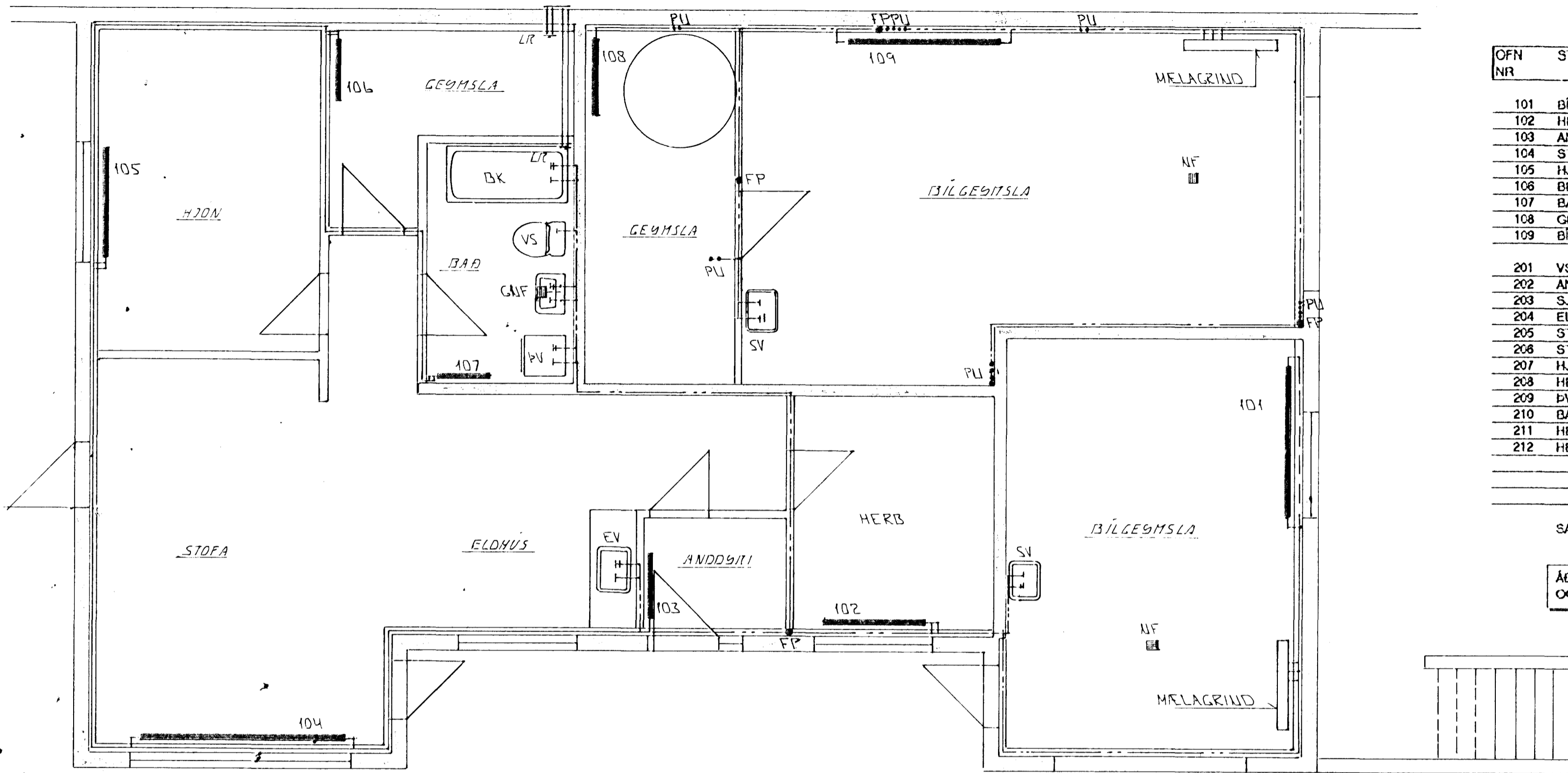
1. HÆÐ GRUNNMÝND. 1:50
