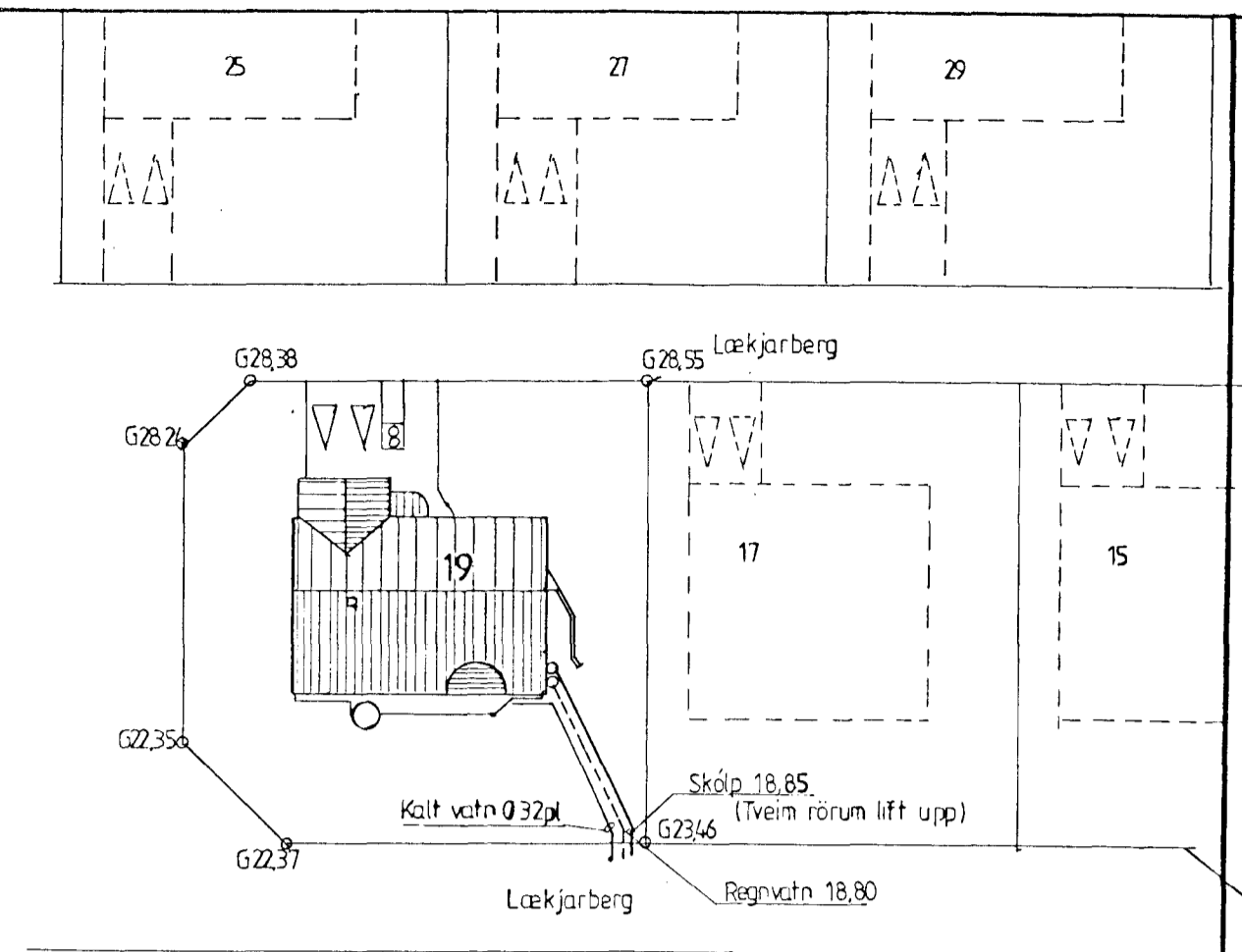
Afstöðumynd 1:500
