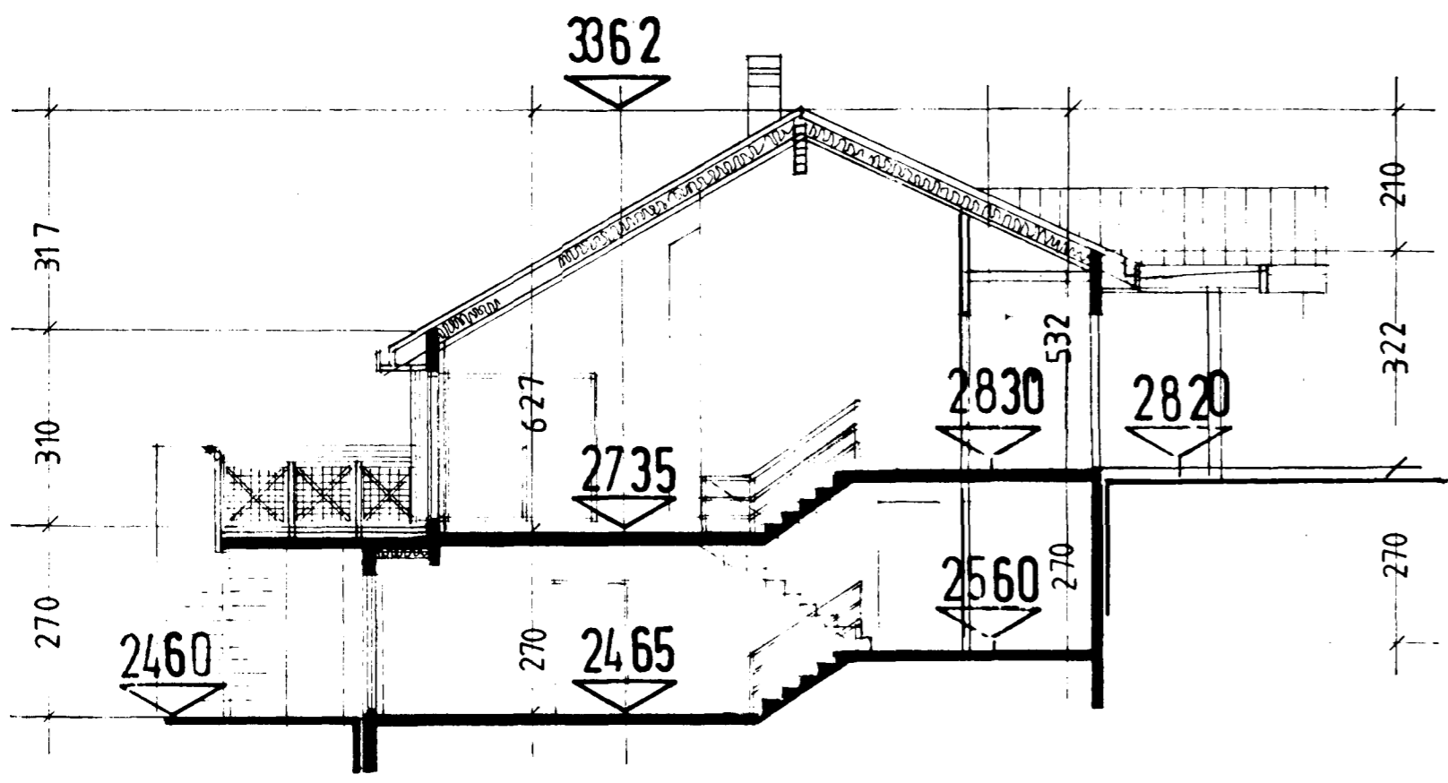
SKURÐUR AA
