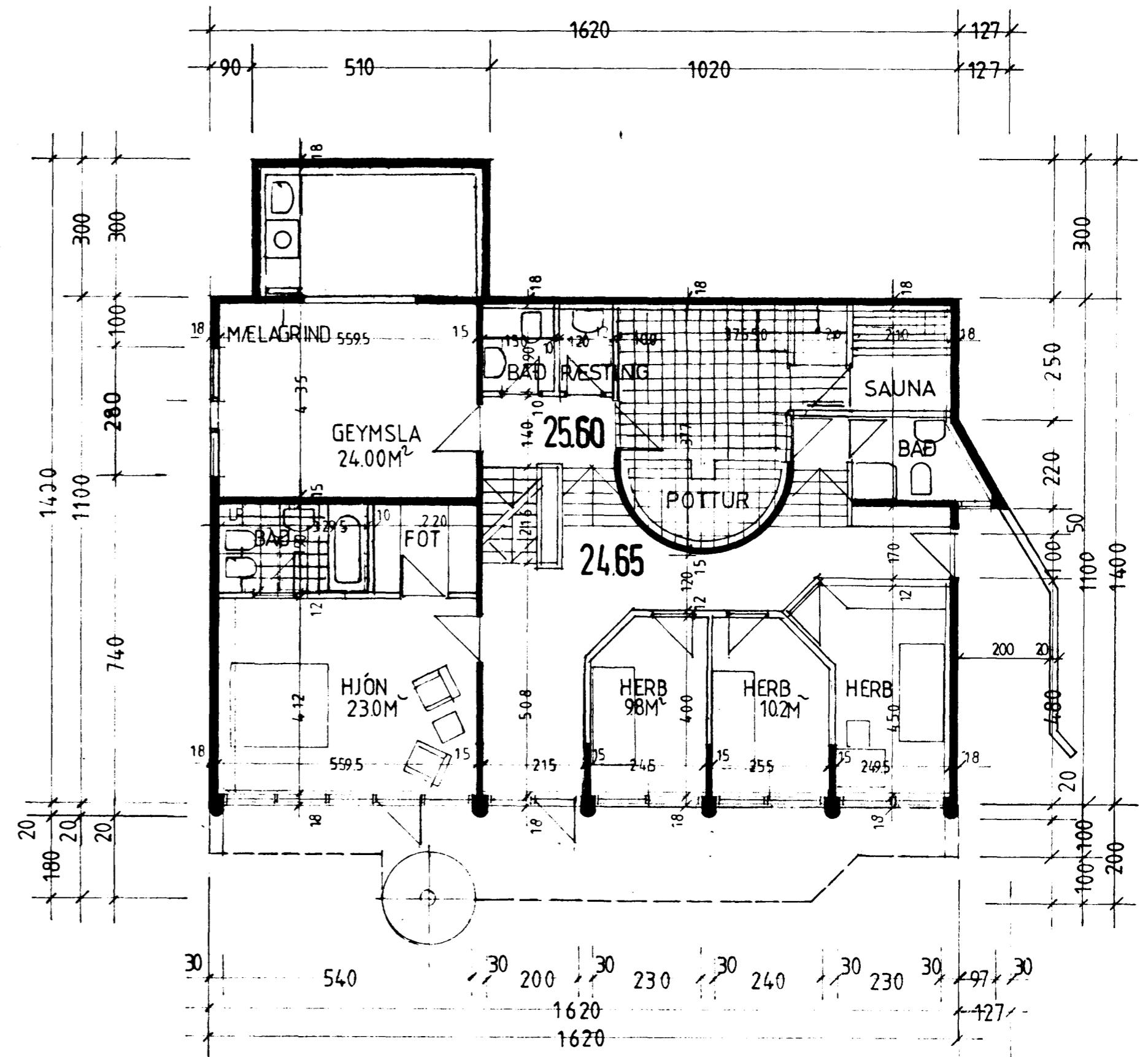
GRUNNMYND KJALLARA
