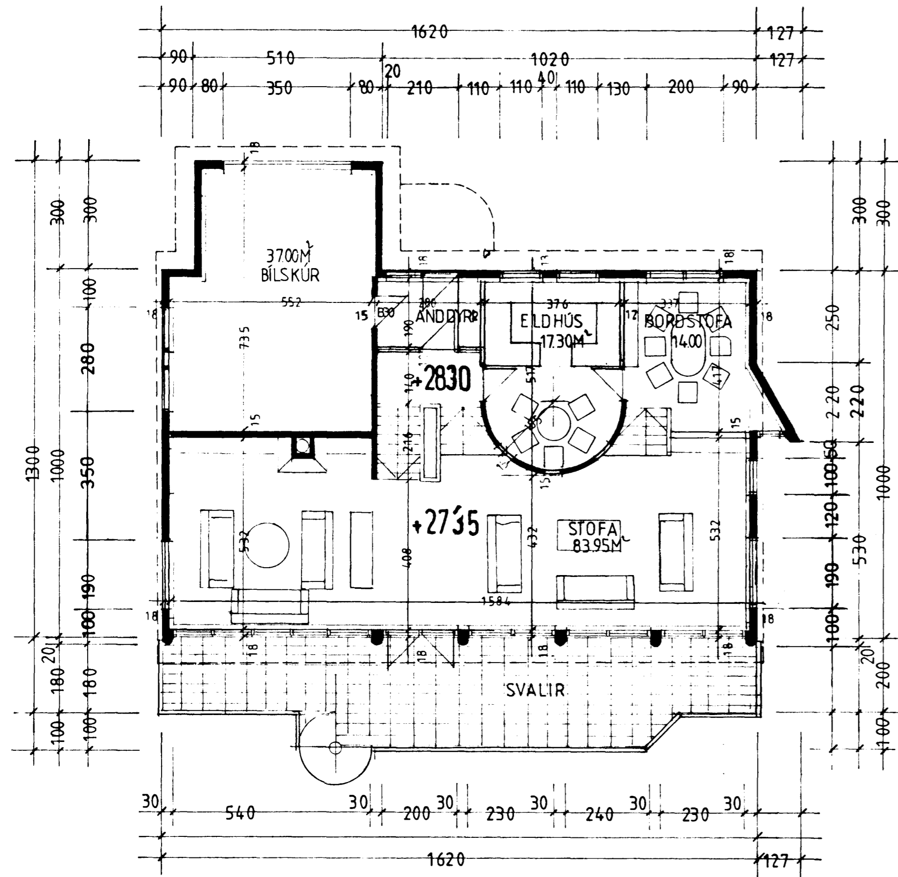
GRUNNMYND JARÐHÆÐAR
