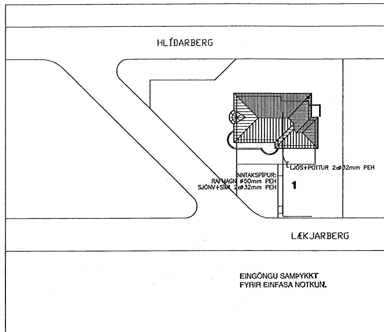
AFSTÖÐUMYND M 1:500
