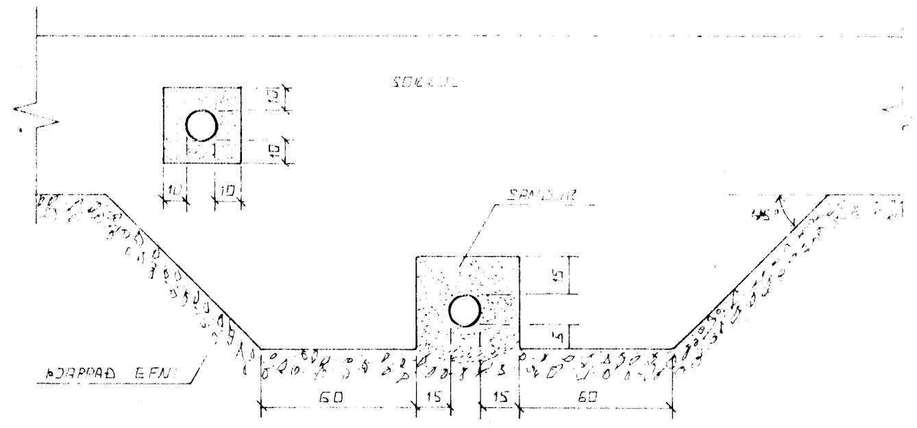
FRÁGANGUR LAGNA UNDIR OG Í SÖKKULVEGG. GRÁFÐ SKAL FÜR LÖGNUM UNDIR SÖKKULUM. AÐUR ER BEIÐ ERU STAFÖÐUR.
