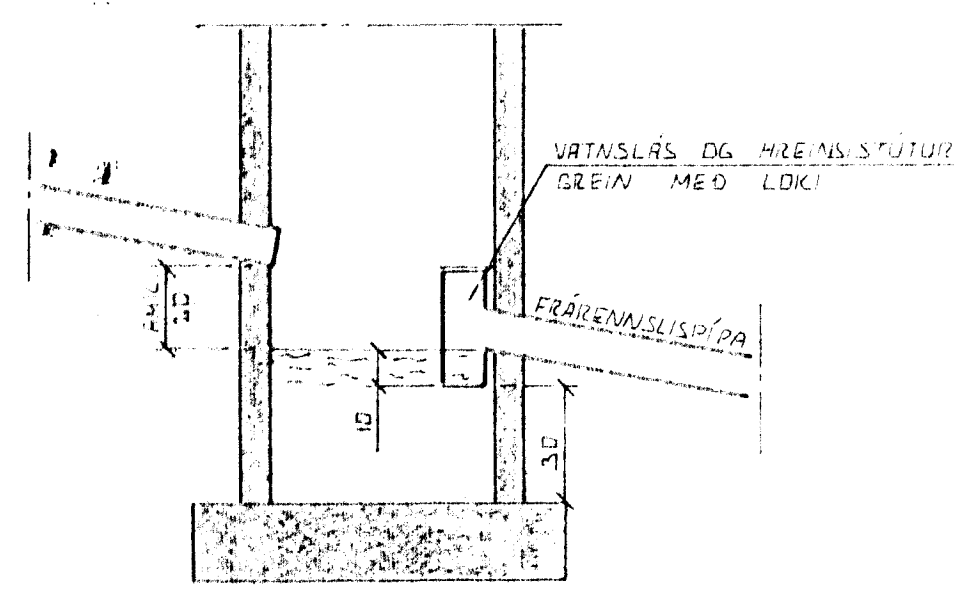
SAFNBRUNNUR BRUNNUR FÜR DÖRVAÐIN OG REIÐVAÐIN FRÆRNISLÍÐIÐ SKAL VEIRA 150 CM FRÓ BEIÐRÖÐI DÖRVEGG.
