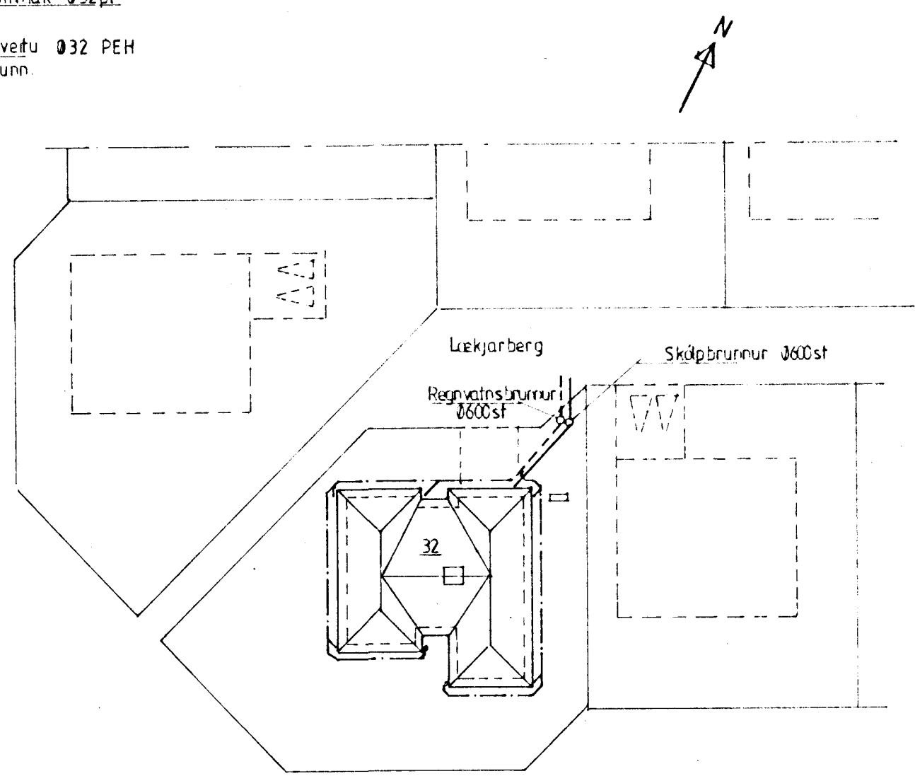
Afstöðumynd 1:500
