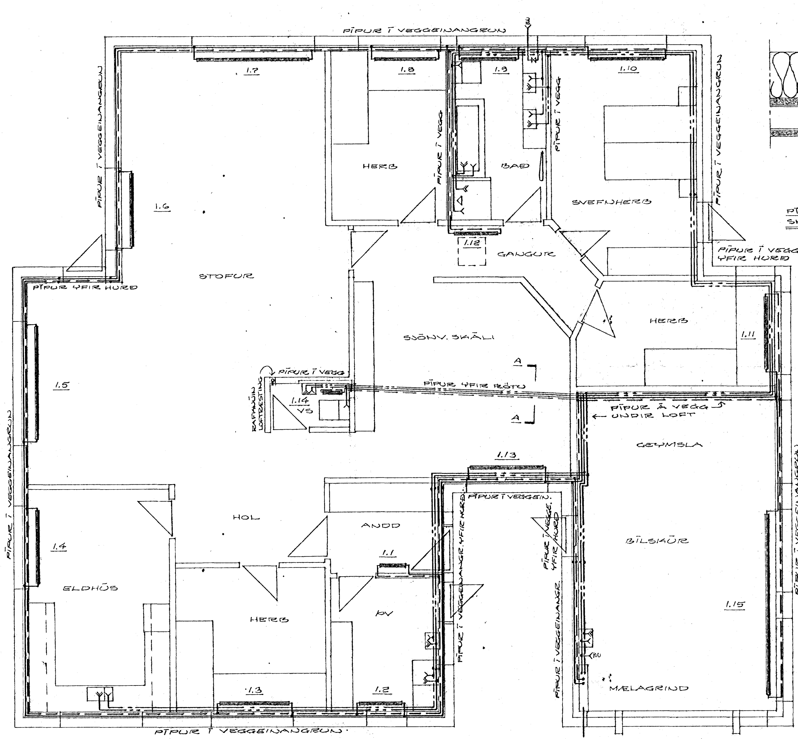
GRUNNMÝND, M=1:150
