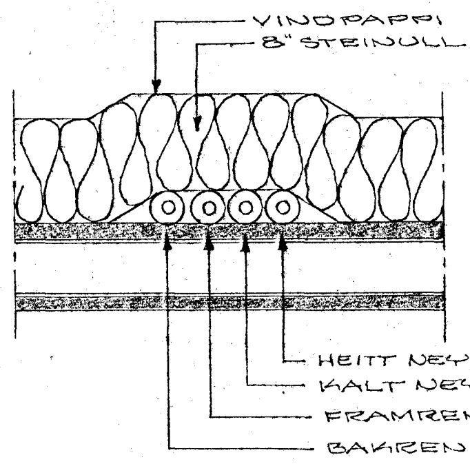
PÍPUR YFIR ÞÉTU SNID A-A, M=1:10
