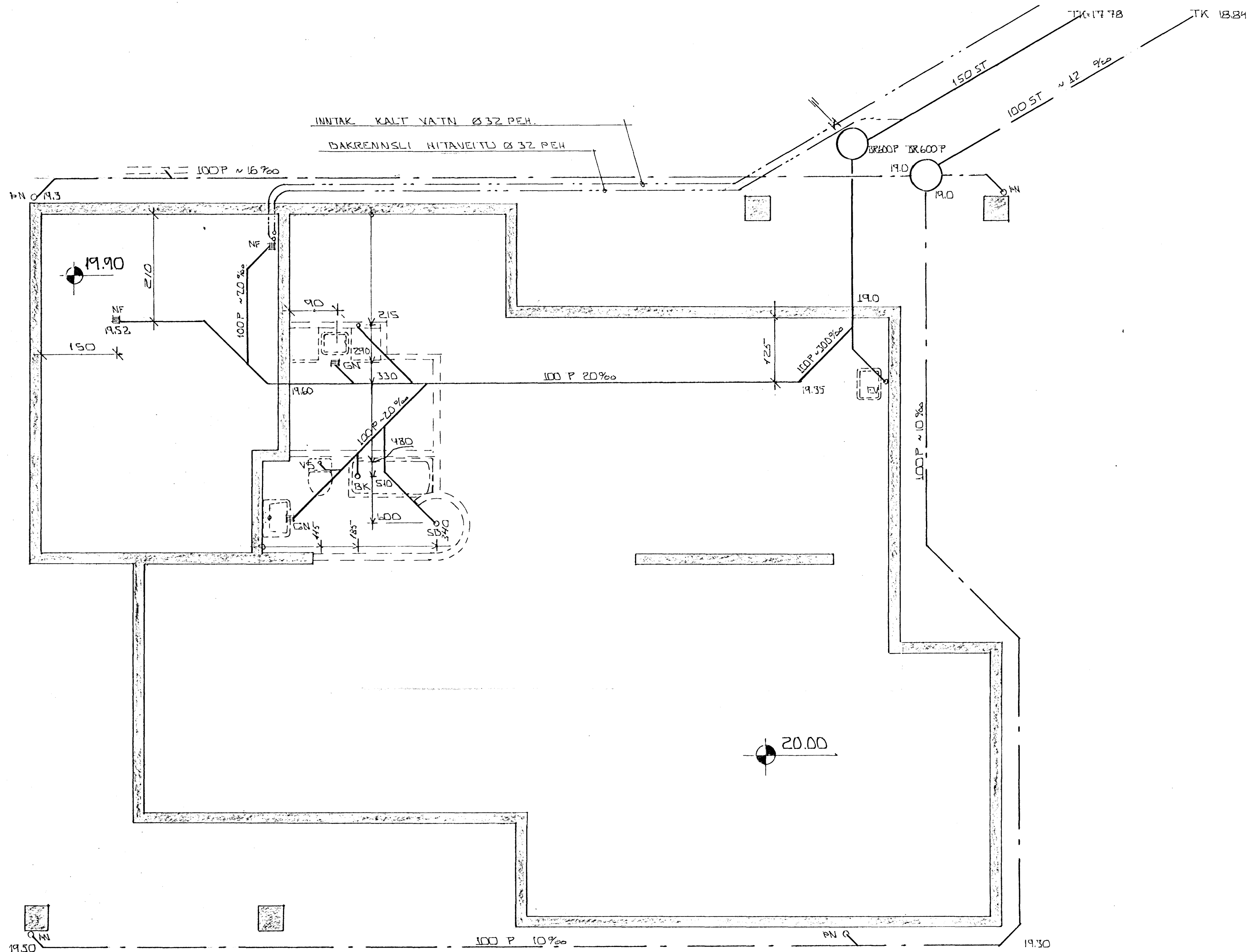
GRUNNMYND 1:50
