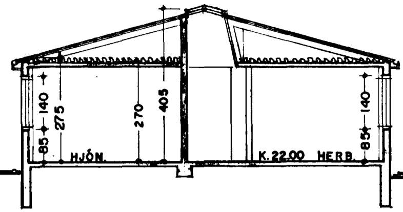
SNEIÐING B - B
