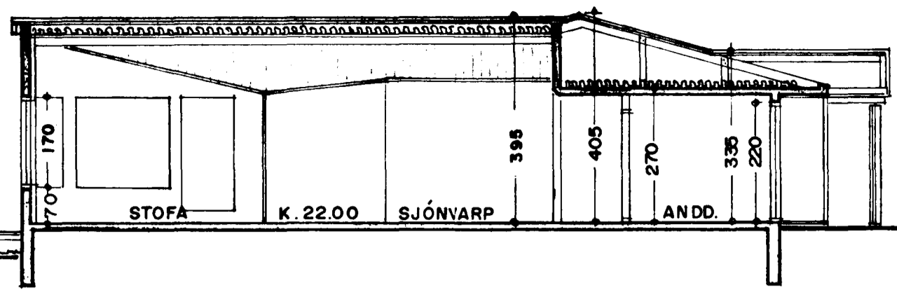
SNEIÐING A - A
