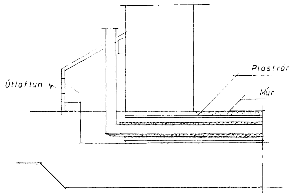
Frágangur í gólf m = 1:5
