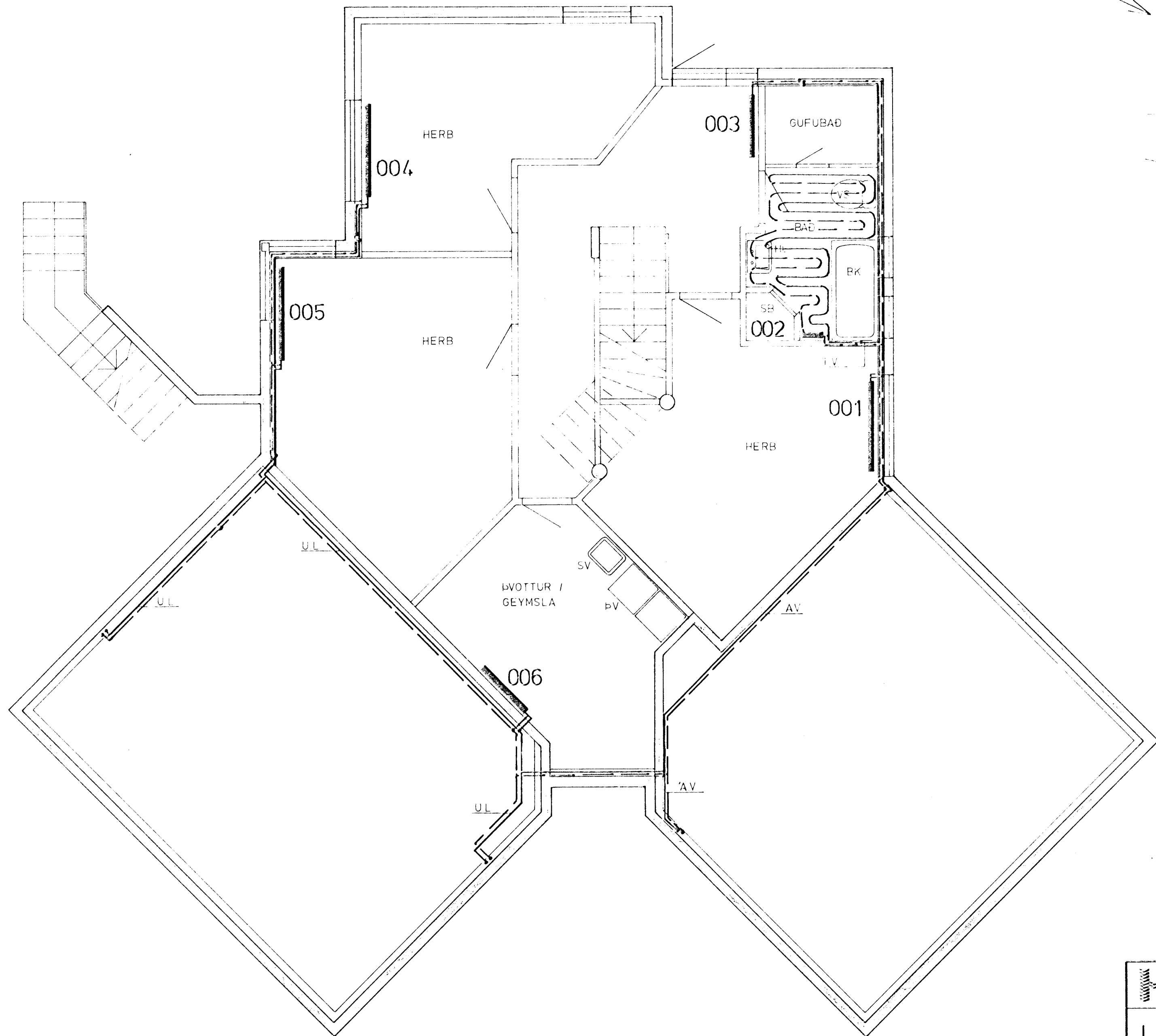
GRUNNMYND NEDRI HÆÐAR 1:50
