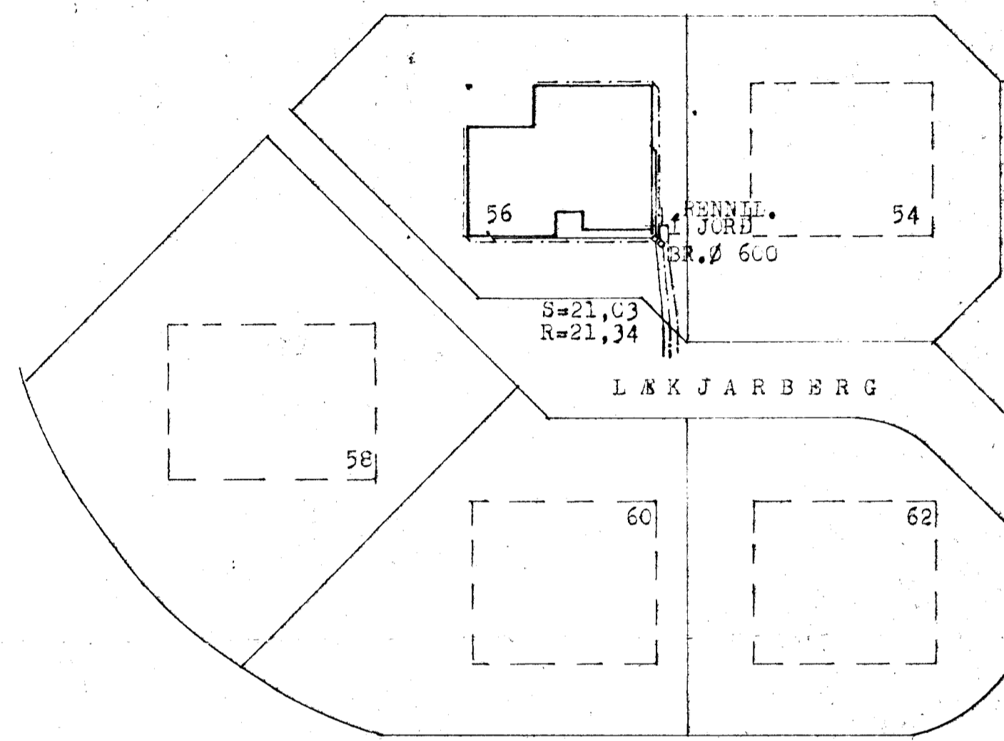
AFSTÖÐUMYND 1:500
