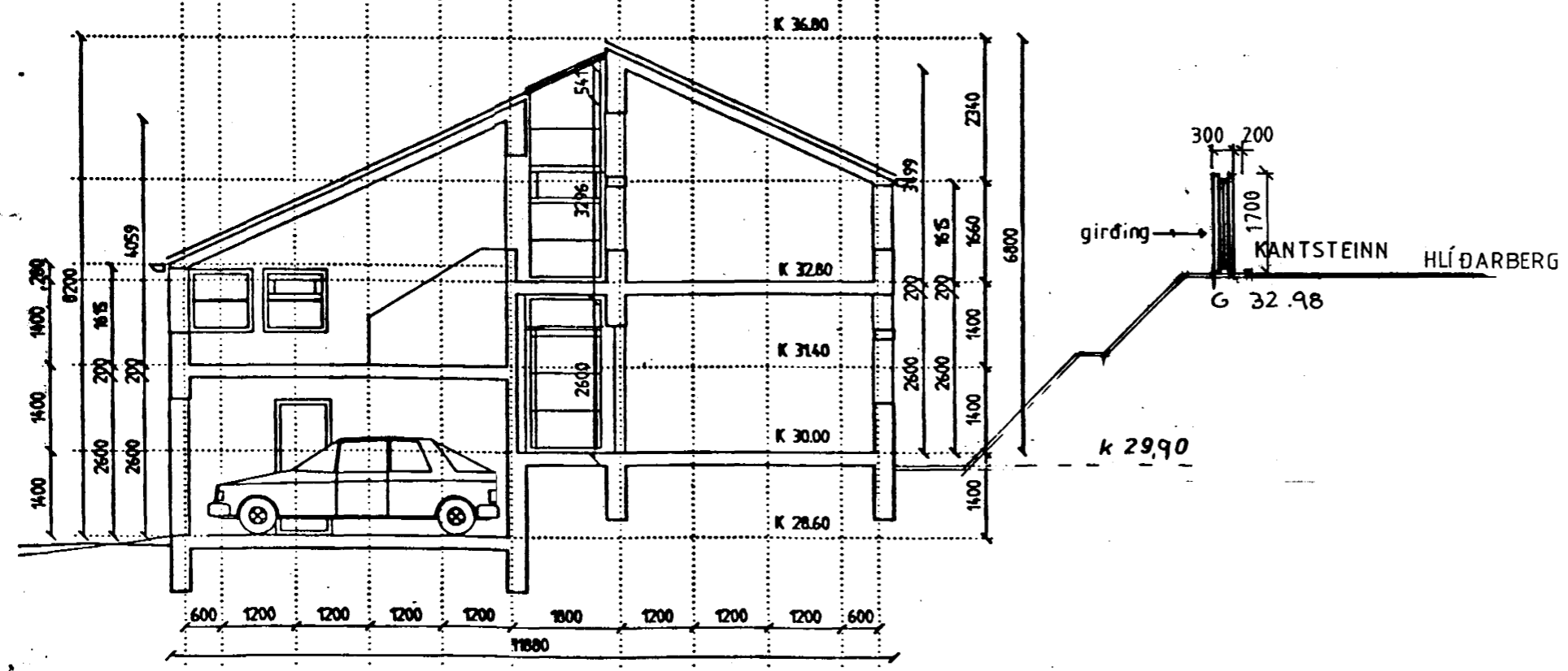
ÞVERSKURÐARMYND B - B
