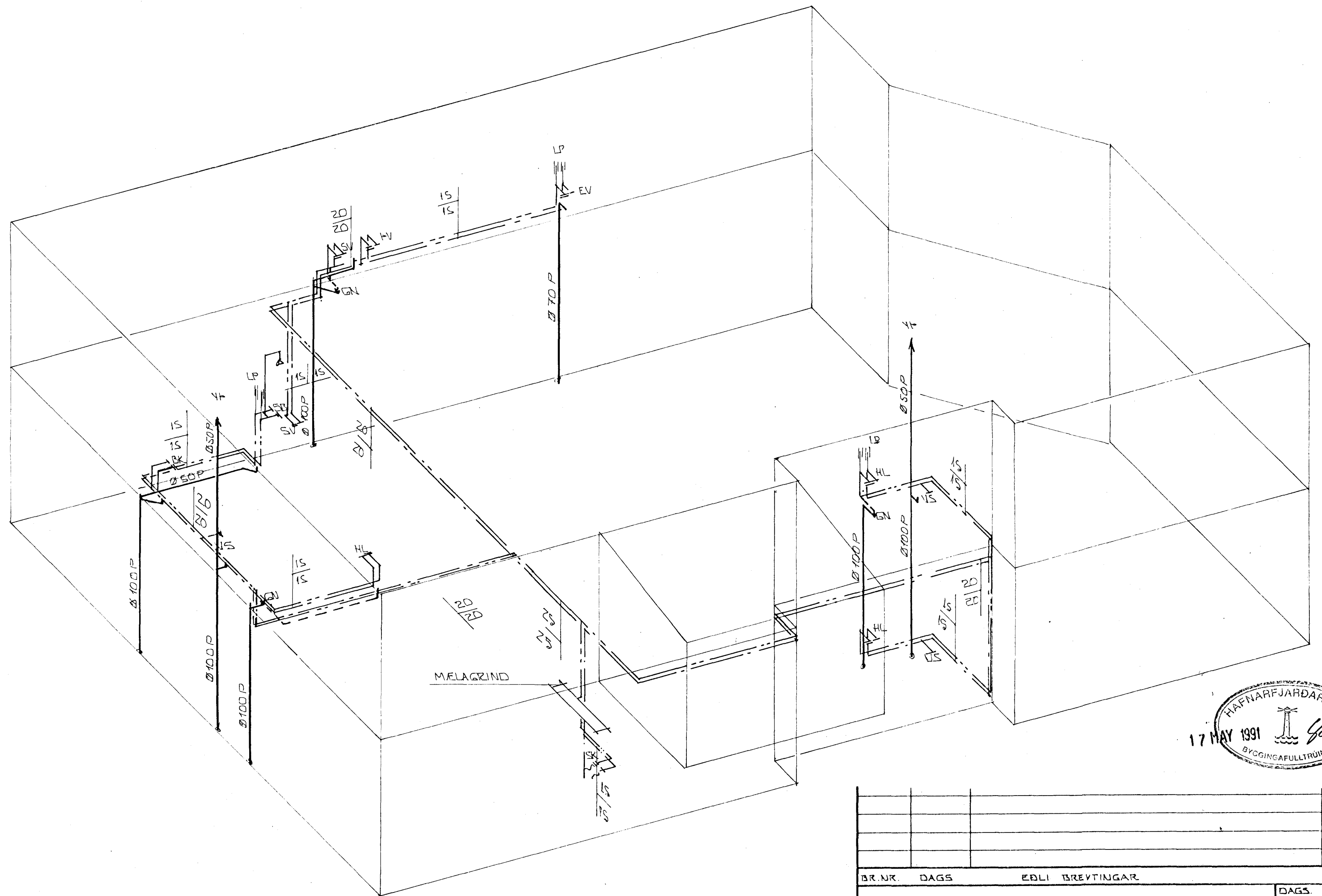
RÚMMYND VATNS- OG FRÆRNNISLISLAGNA 1:50
