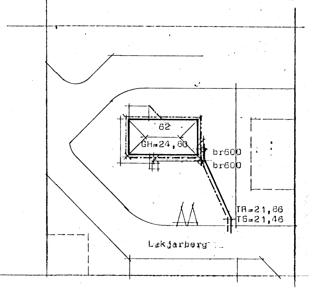
Afstöðumynd Mk 1:500
