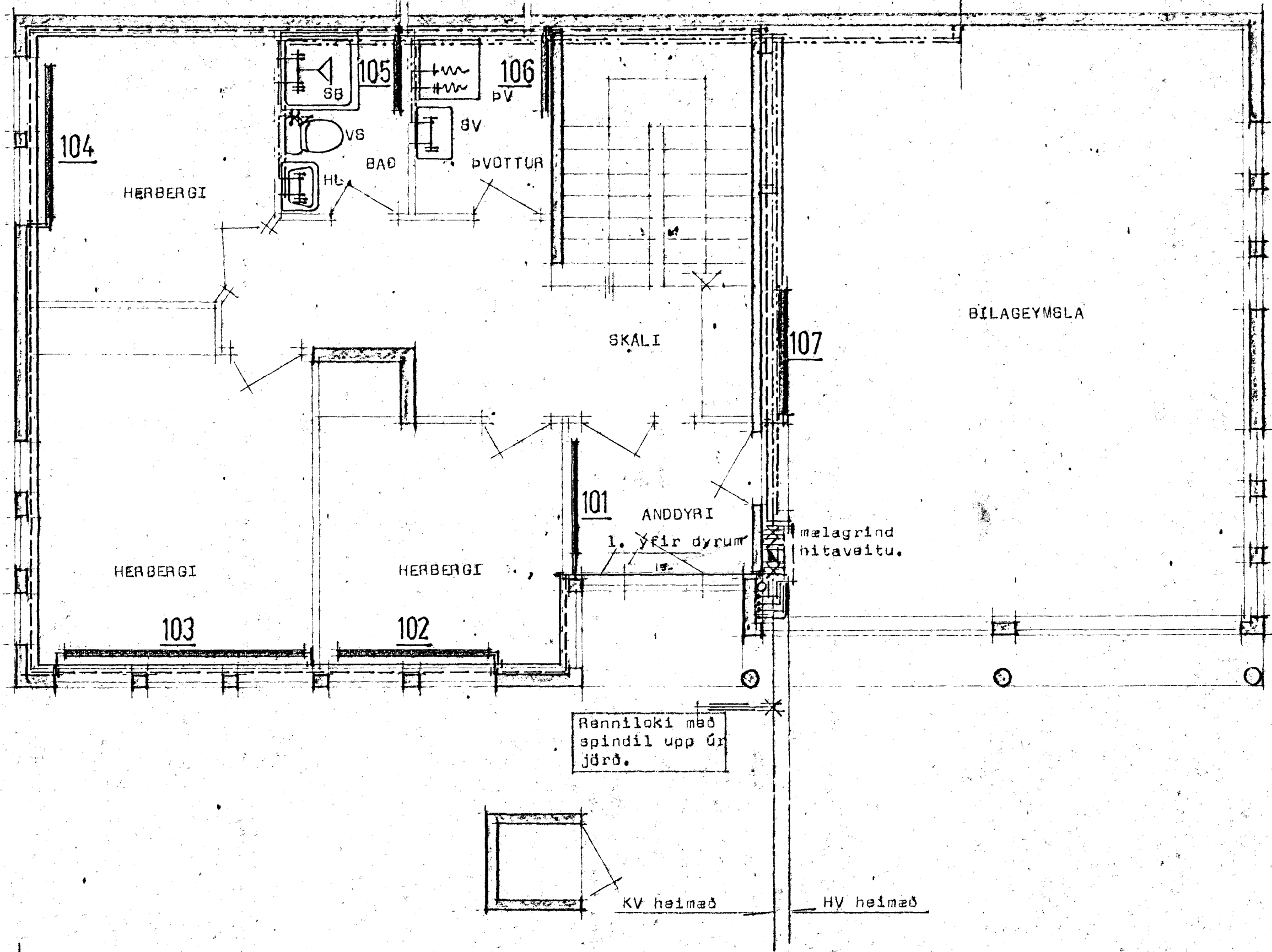
Grunnmynd neðri hæðar MK 1:50
