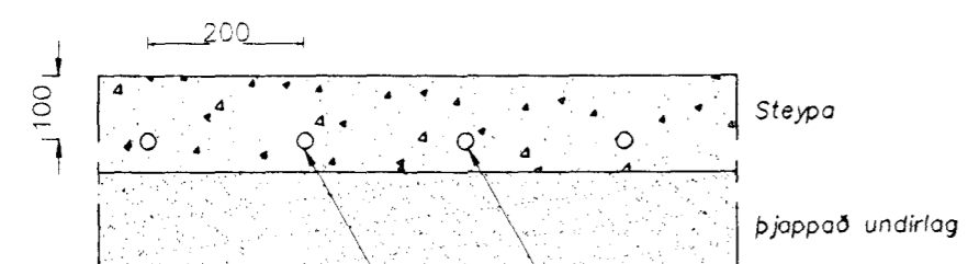
Ø20 PEX rör hitapólin fest við jöfnagrind í steyptri plötu
