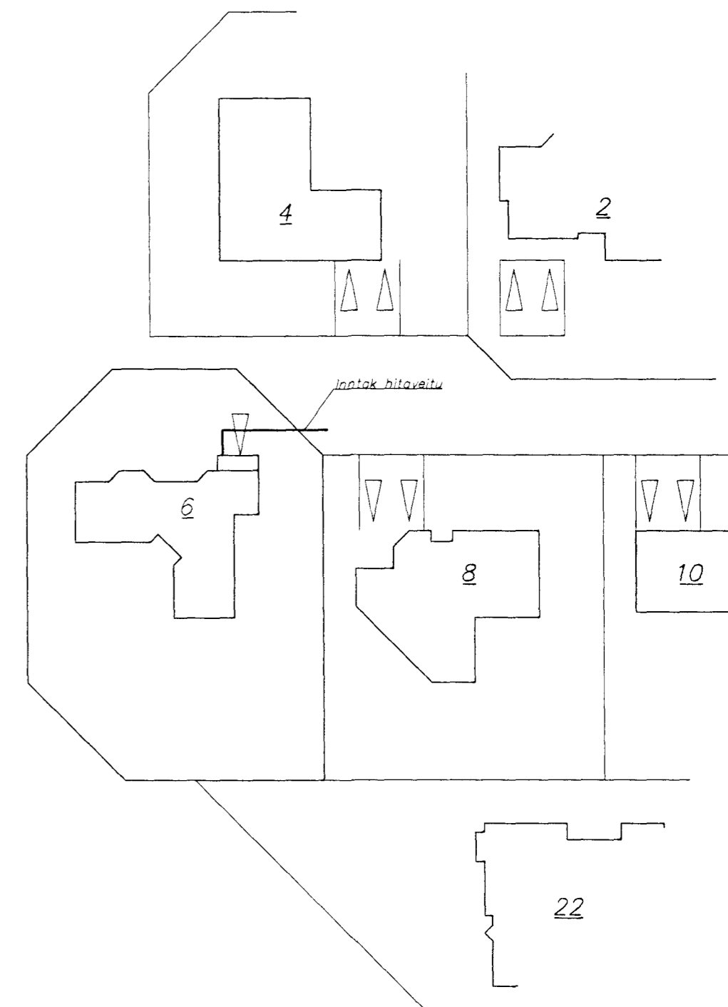
Afstöðumynd 1:500
