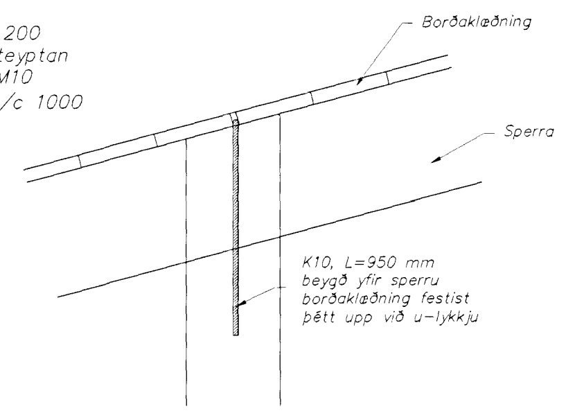
Sperrufesting í steypnan vegg 1:10
