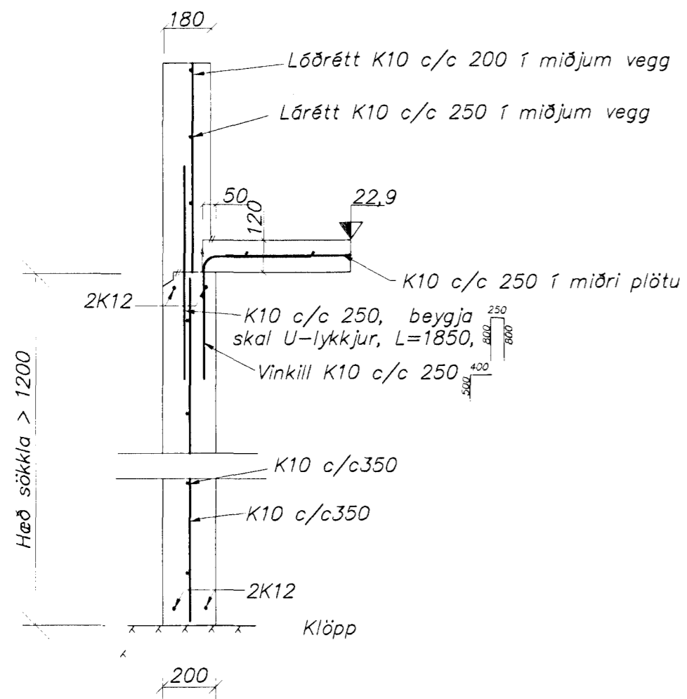
Snið A-A 1:20
