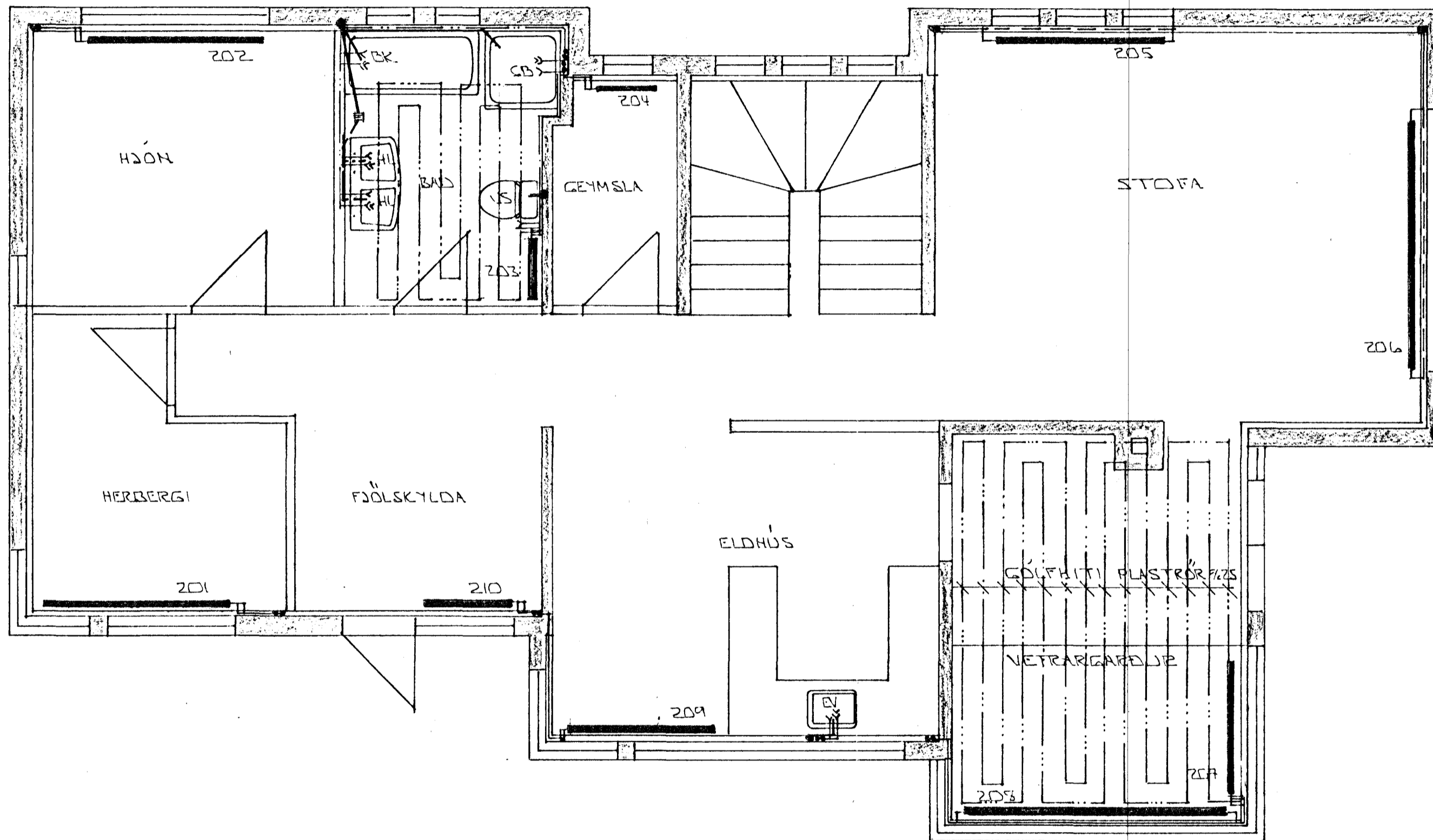
GRUNNMÝND 2. HÆÐ 1:50
