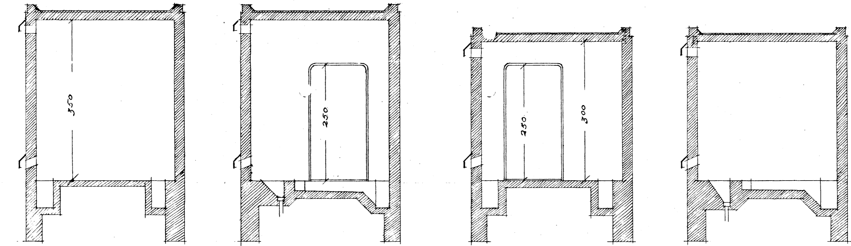
Sníð A-A
