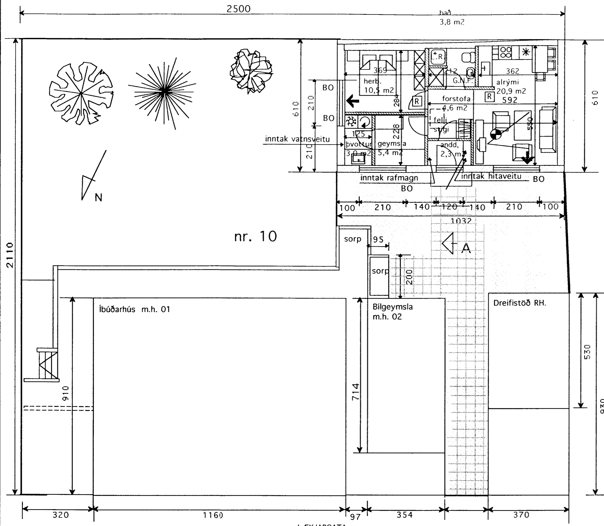
GRUNNMYND 1:100
