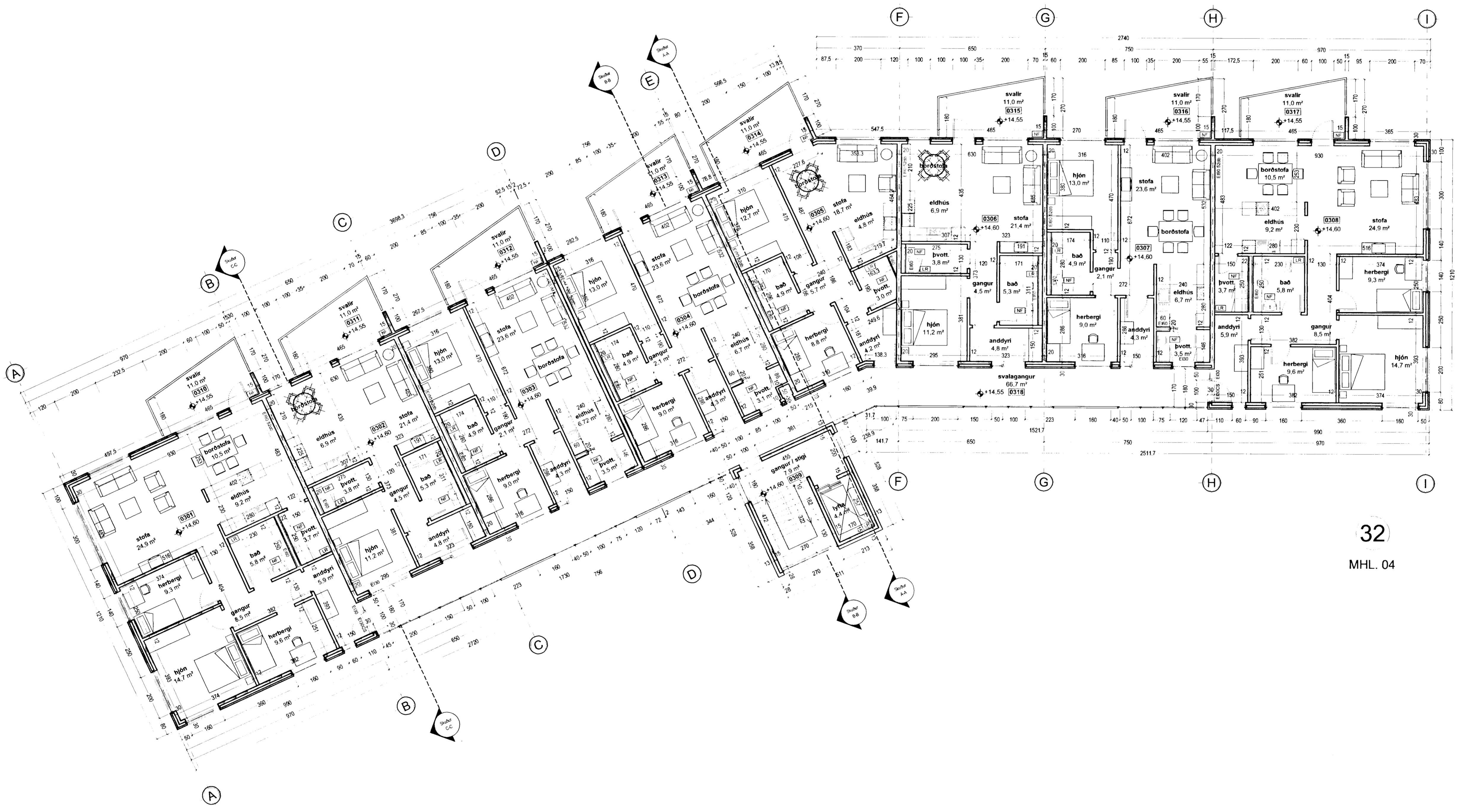
grunnmynd 3.hæð
