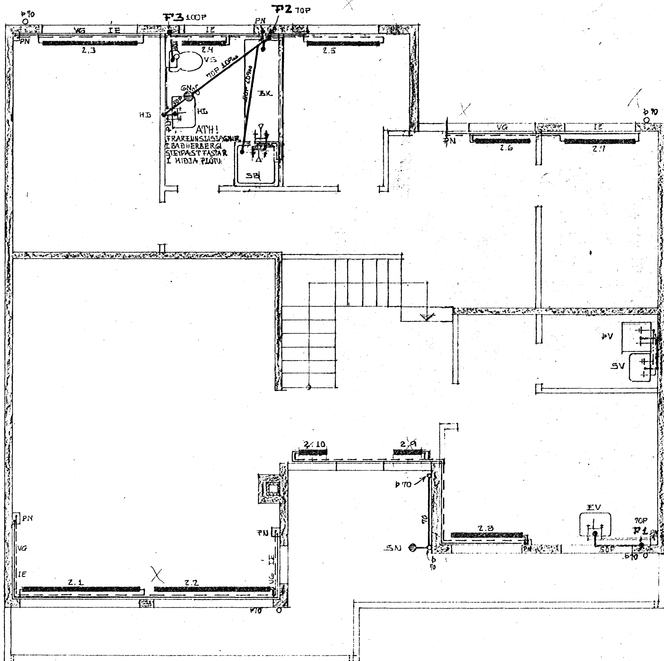
GRUNNMYND 1:50
