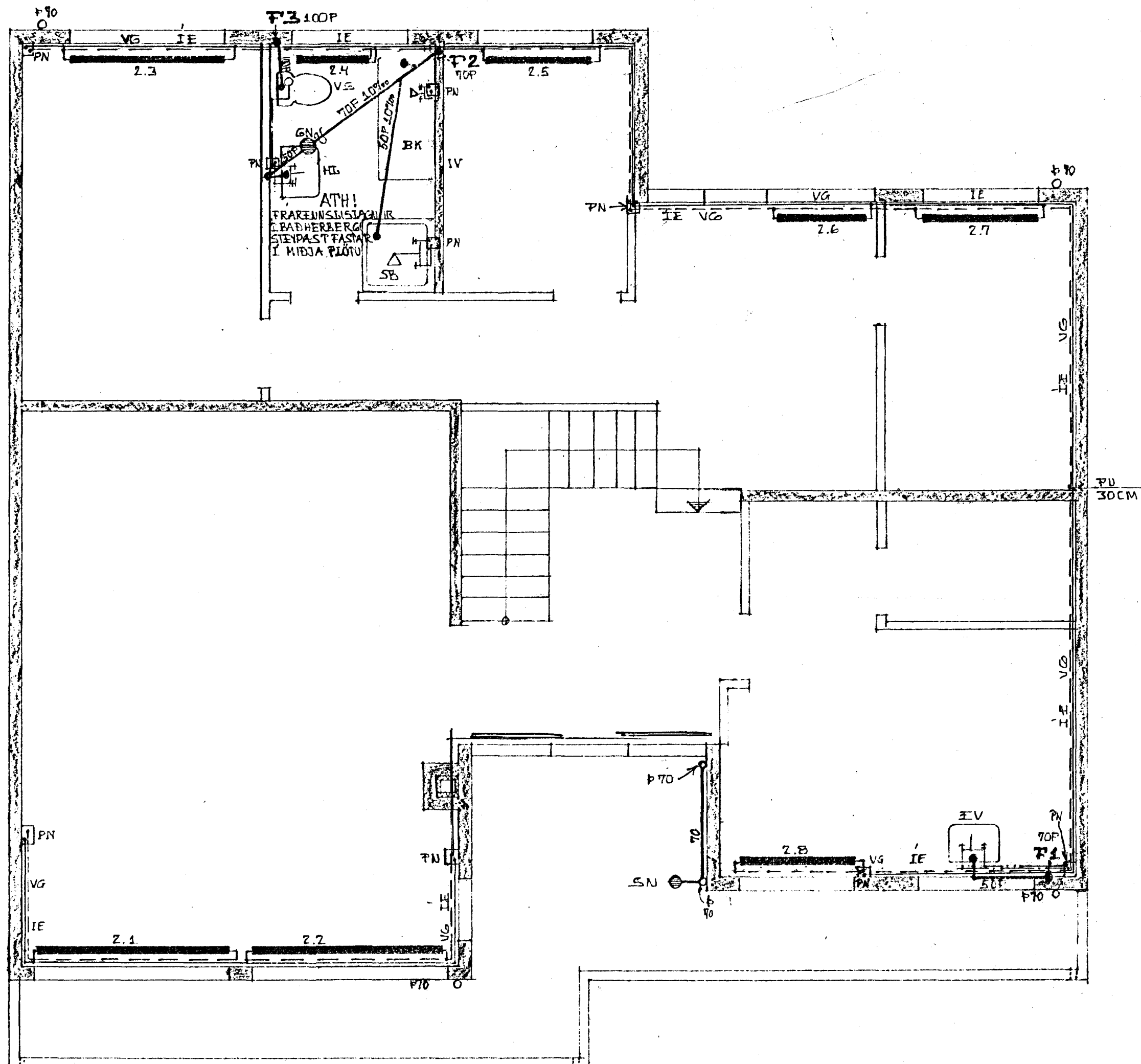
GRUNNMYND 1:50
