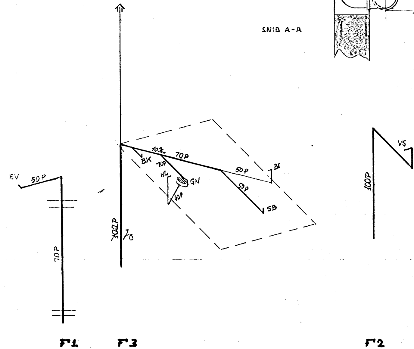
KERTISMUNDIR FRÆNNISLAGNARNA 1:50
