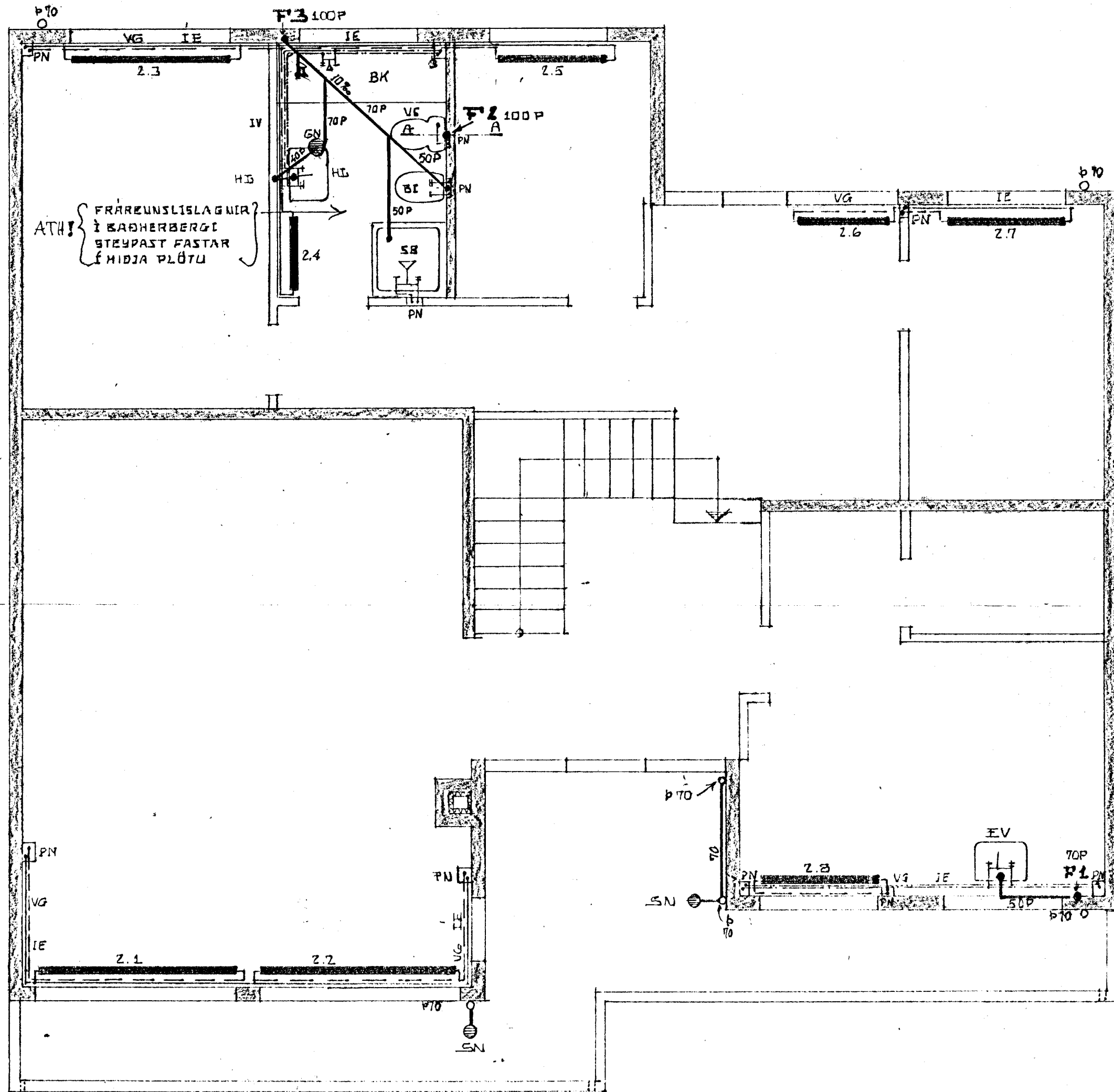
GRUNNMYND 1:50
