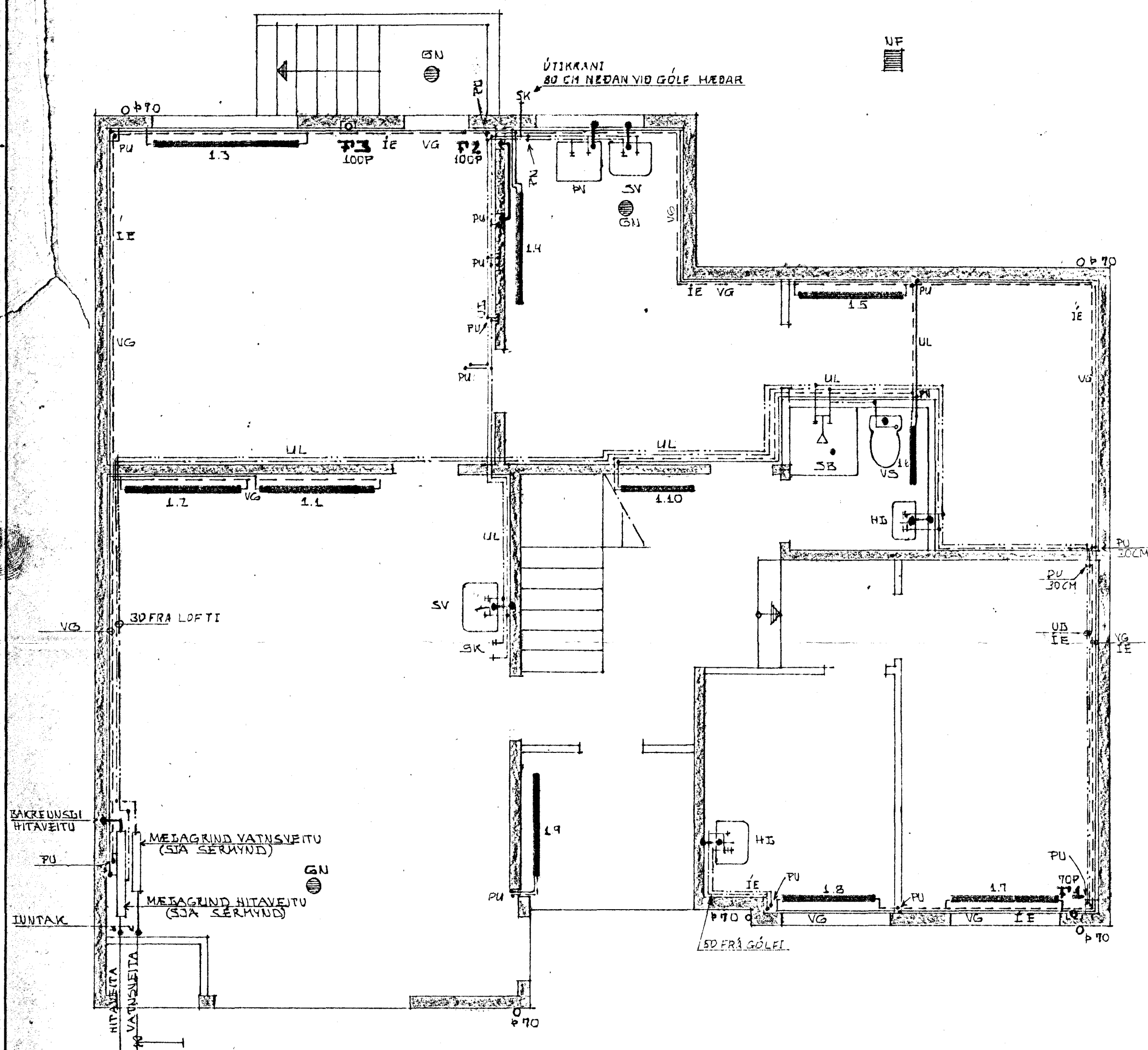
GRUNNMYND 1:50
