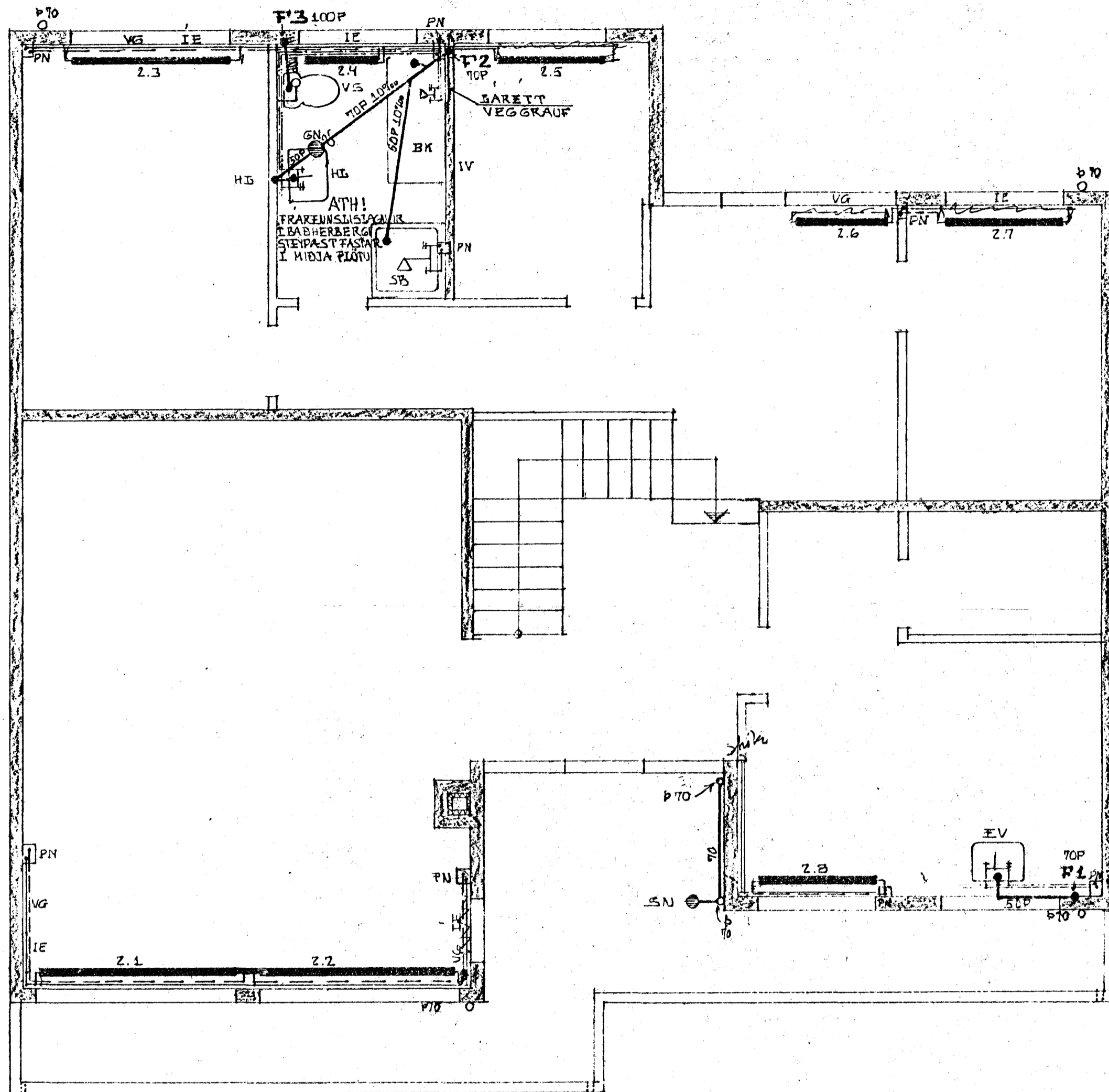
GRUNNMYND 1:50
