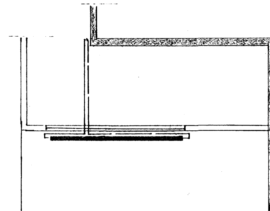
RISHÆÐ 1:50.
