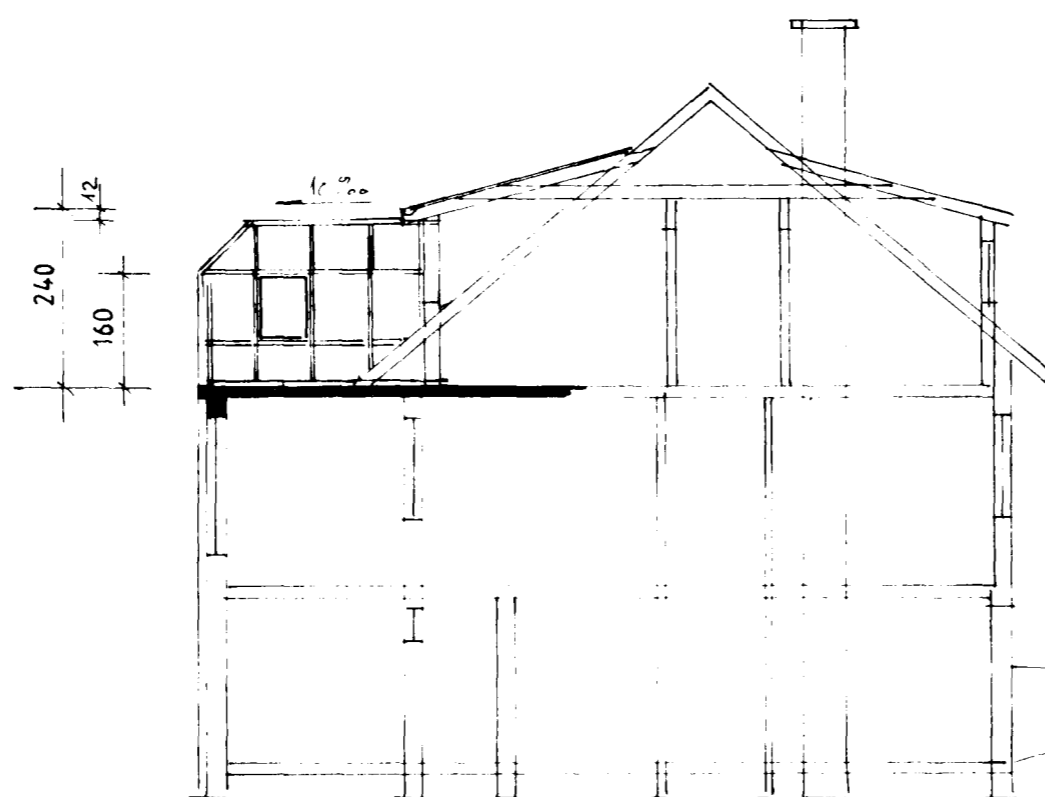
SKURÐUR
