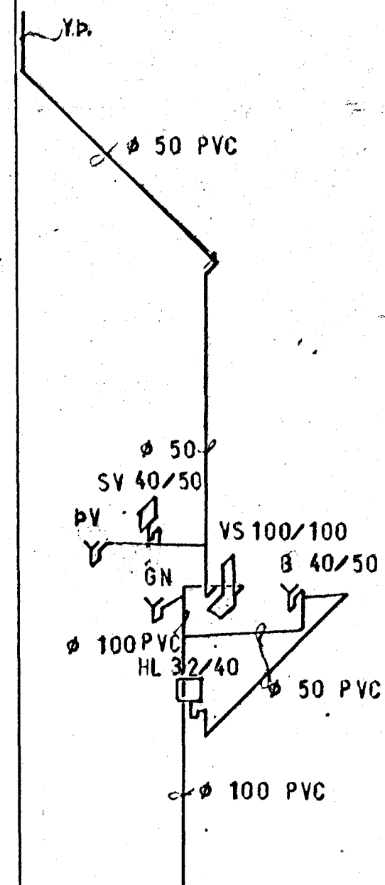
KERFI 1:50
