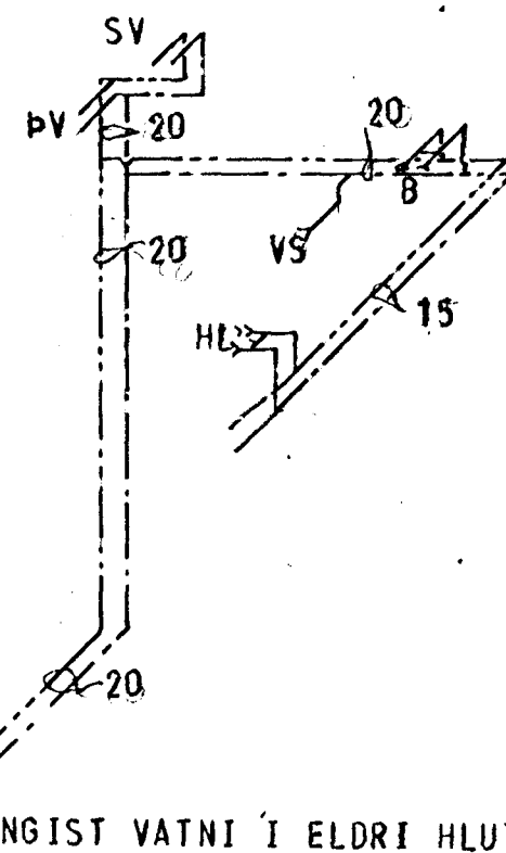
KERFI 1 : 50
