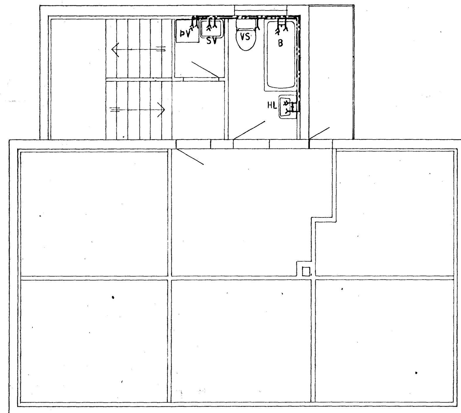
GRUNNMYND 1 : 50
