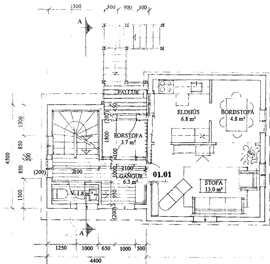
GRUNNMYND 1. HÆÐ
