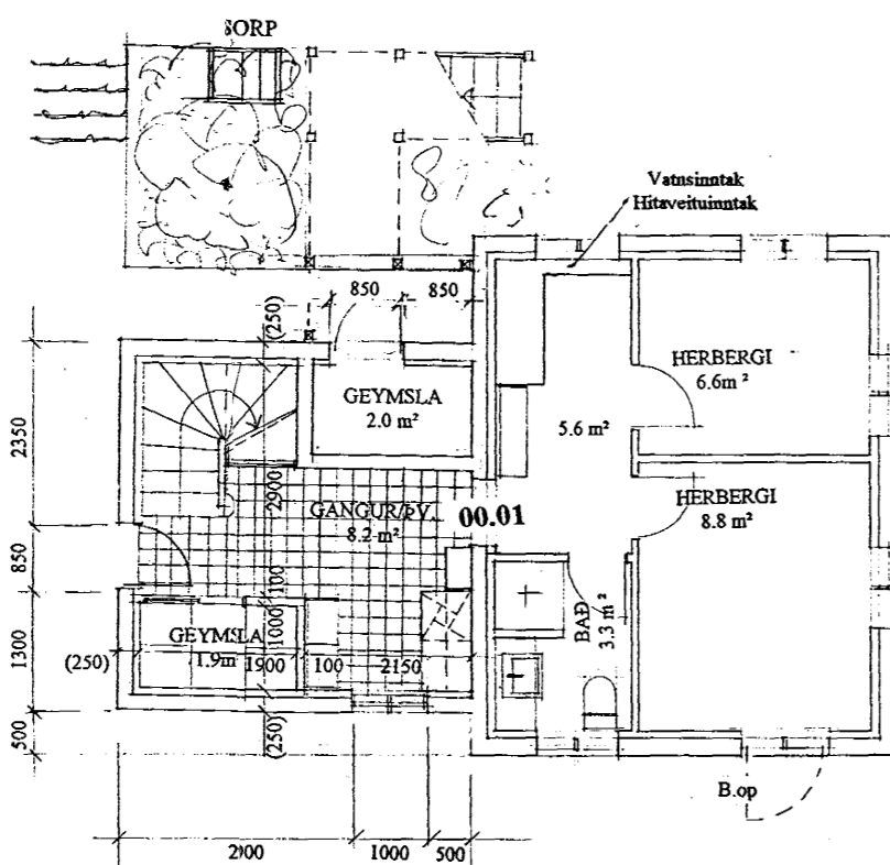
GRUNNMYND KJALLARA
