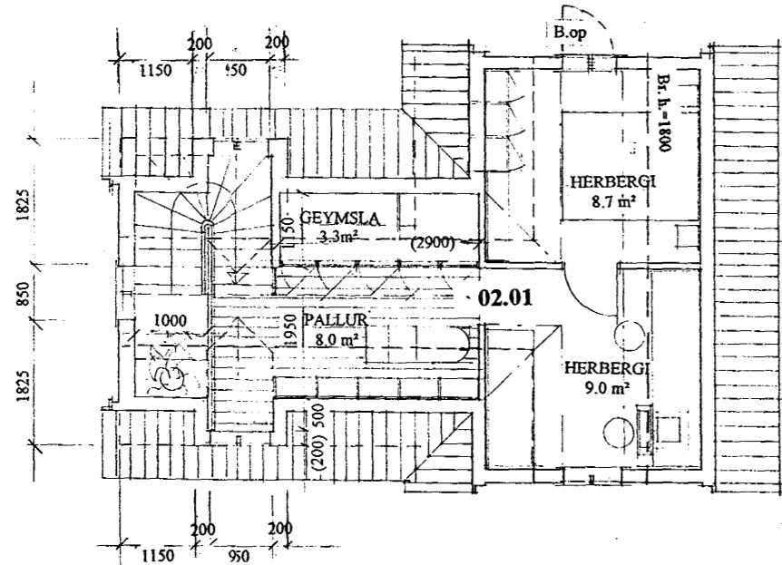
GRUNNMYND 2. HÆÐ
