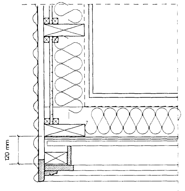
SNEIÐING I VINDSKED A GAFLI
