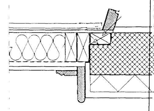
SNEIÐING I VEGG VED TRÖPPU
