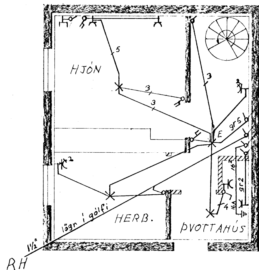
1 hæð
