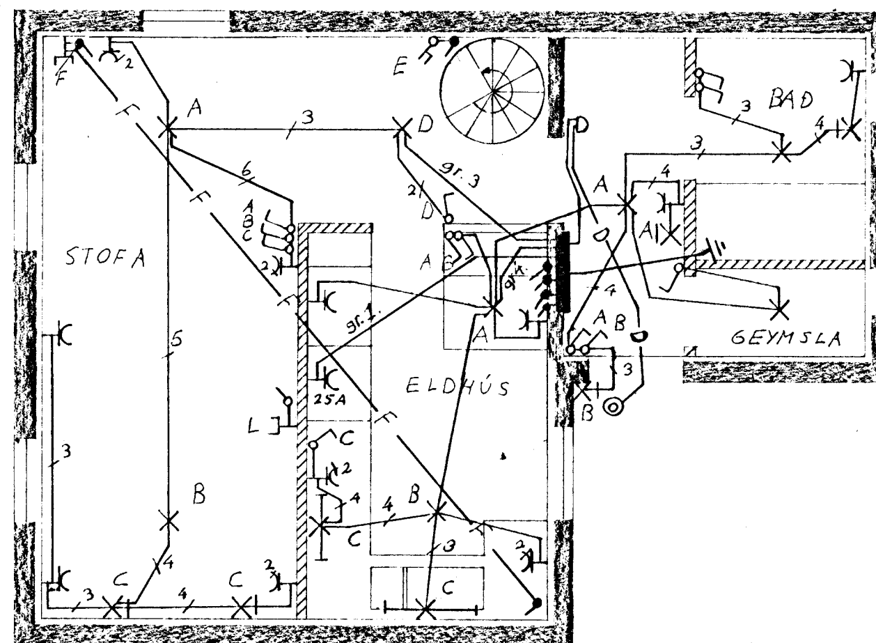
2 hæð
