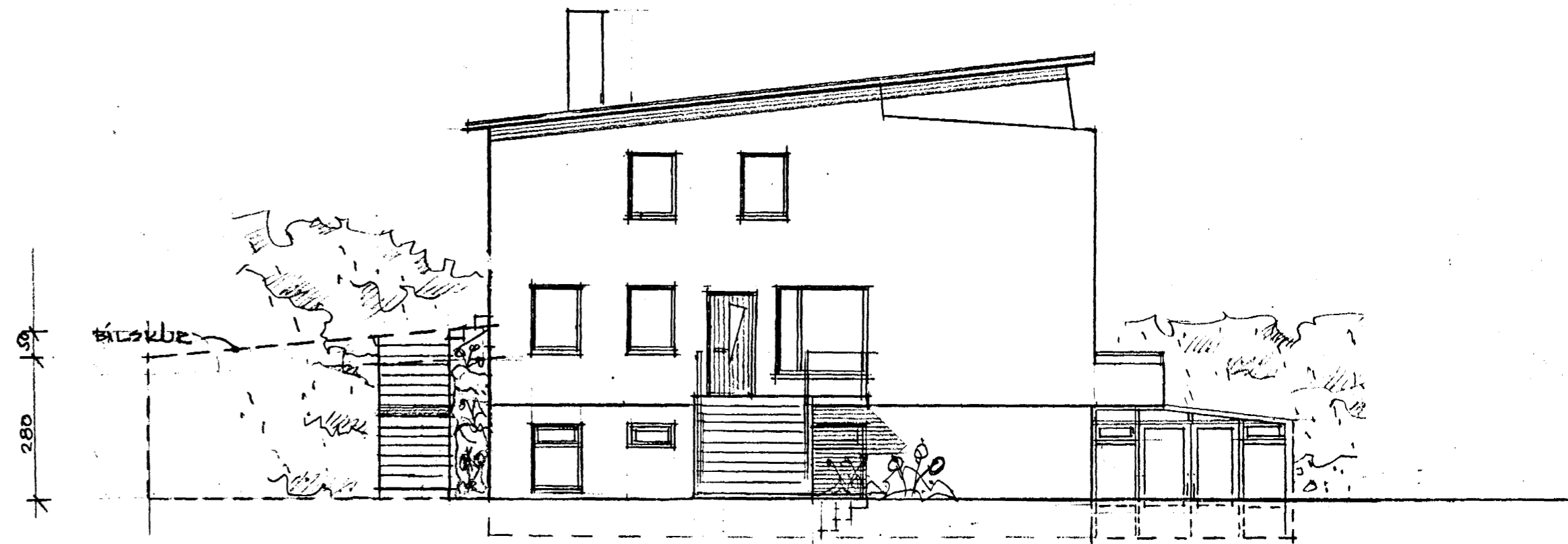
NORÐVESTUR 1:100
