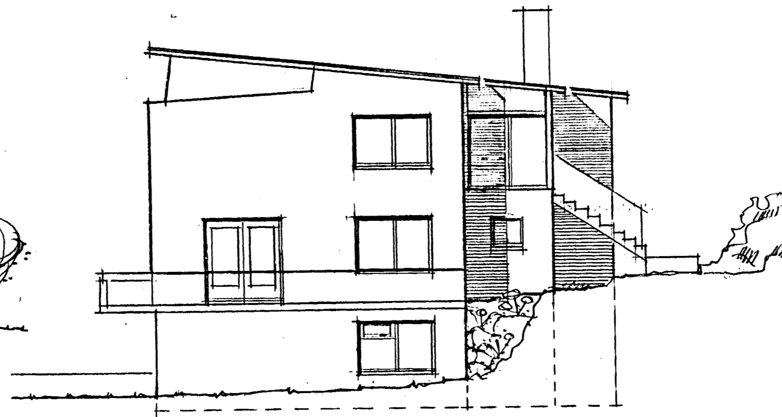
SUÐAUSTUR 1:100
