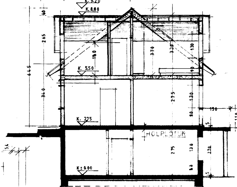
SNÍÐ M. 1:100
