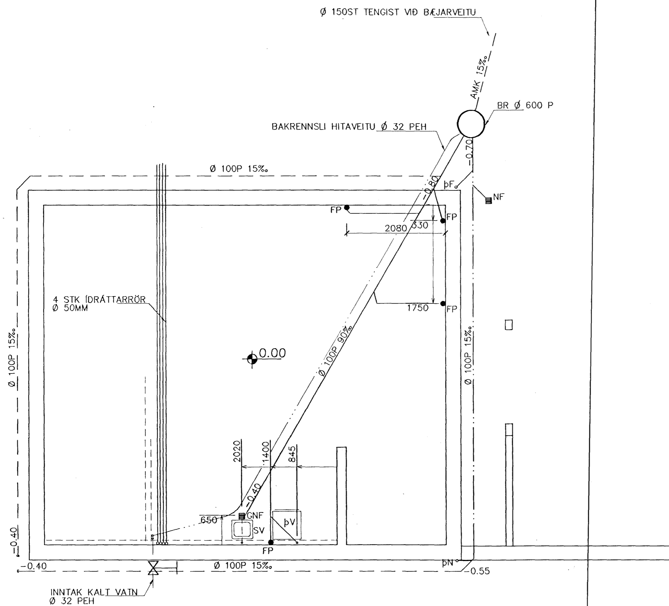
GRUNNMYND 1:50
