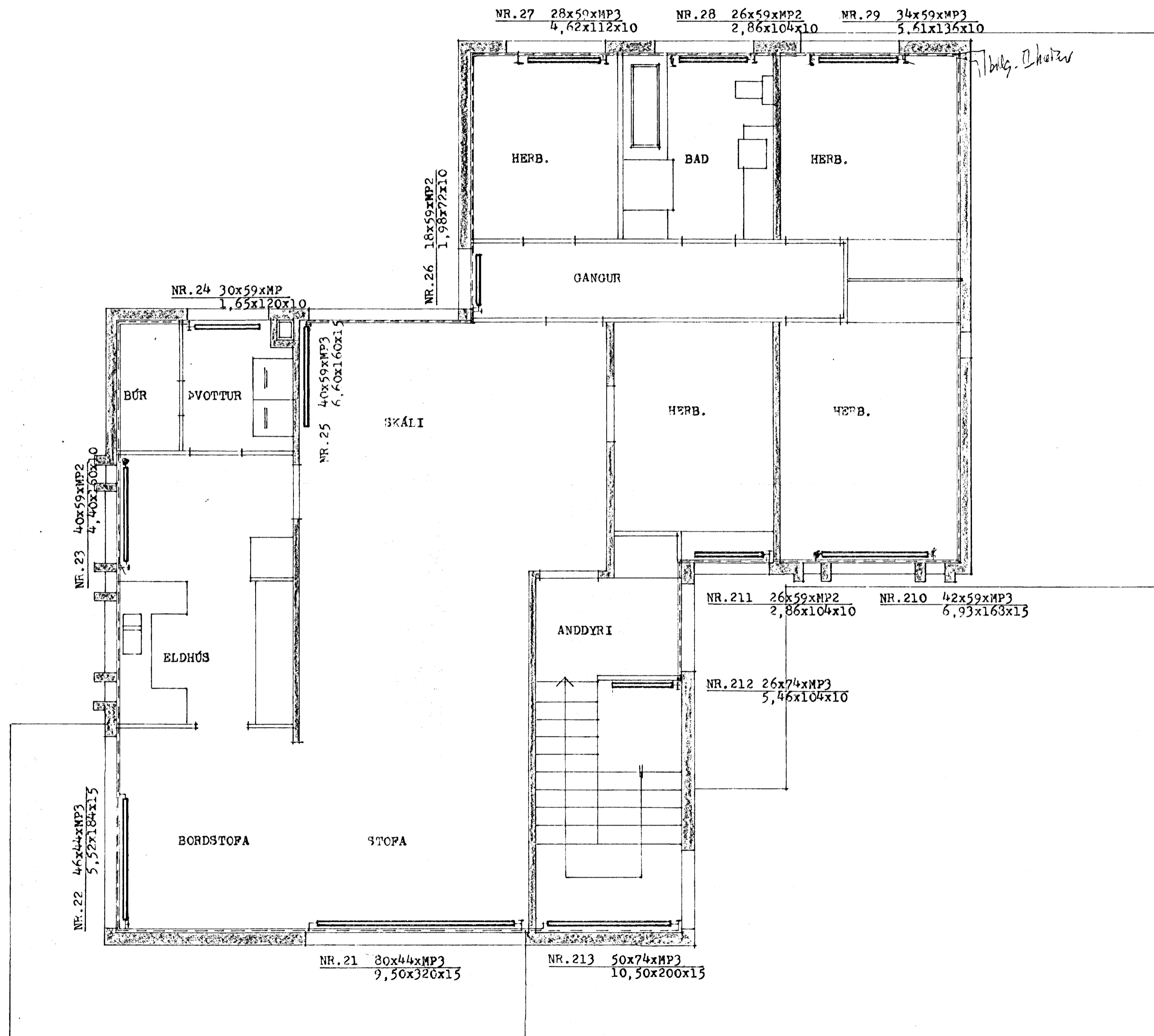
2. HÆÐ GRUNNMYND
