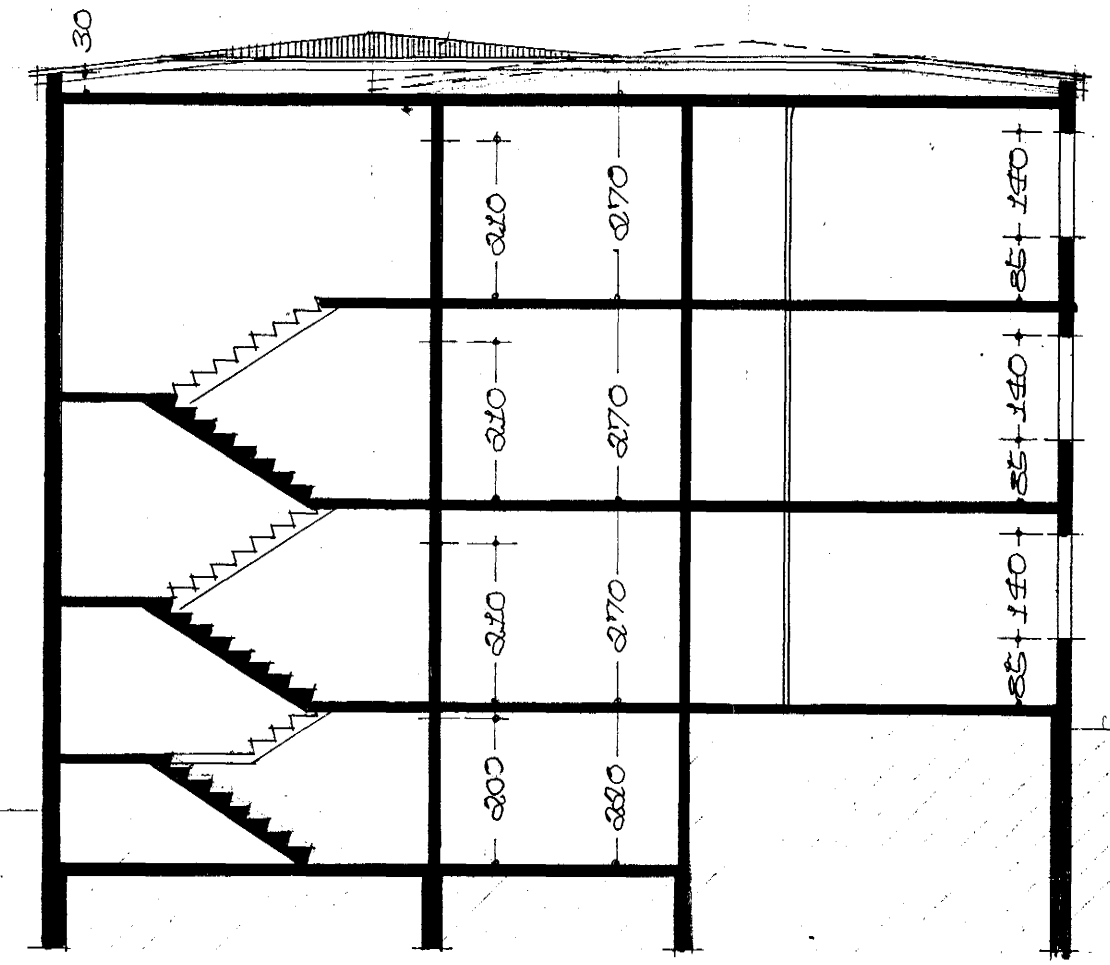
SKURÐUR A-A
