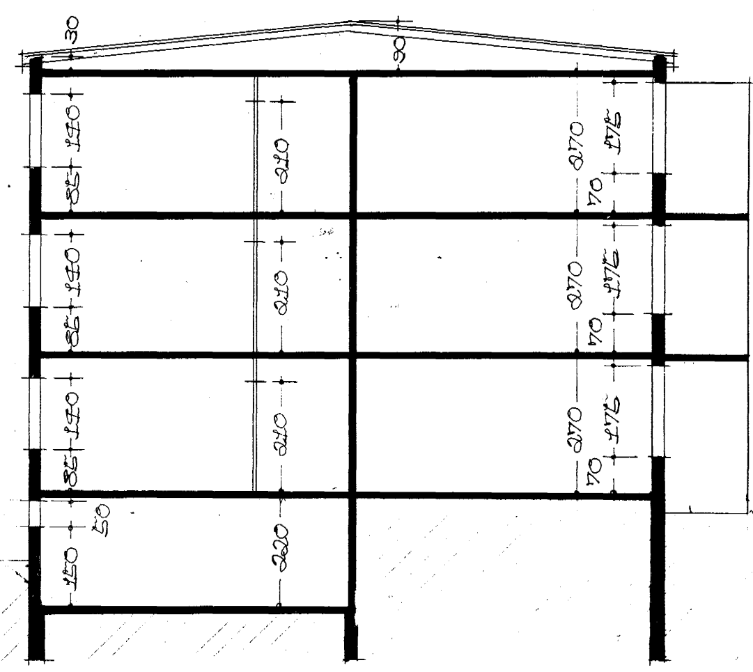
SKURÐUR B-B
