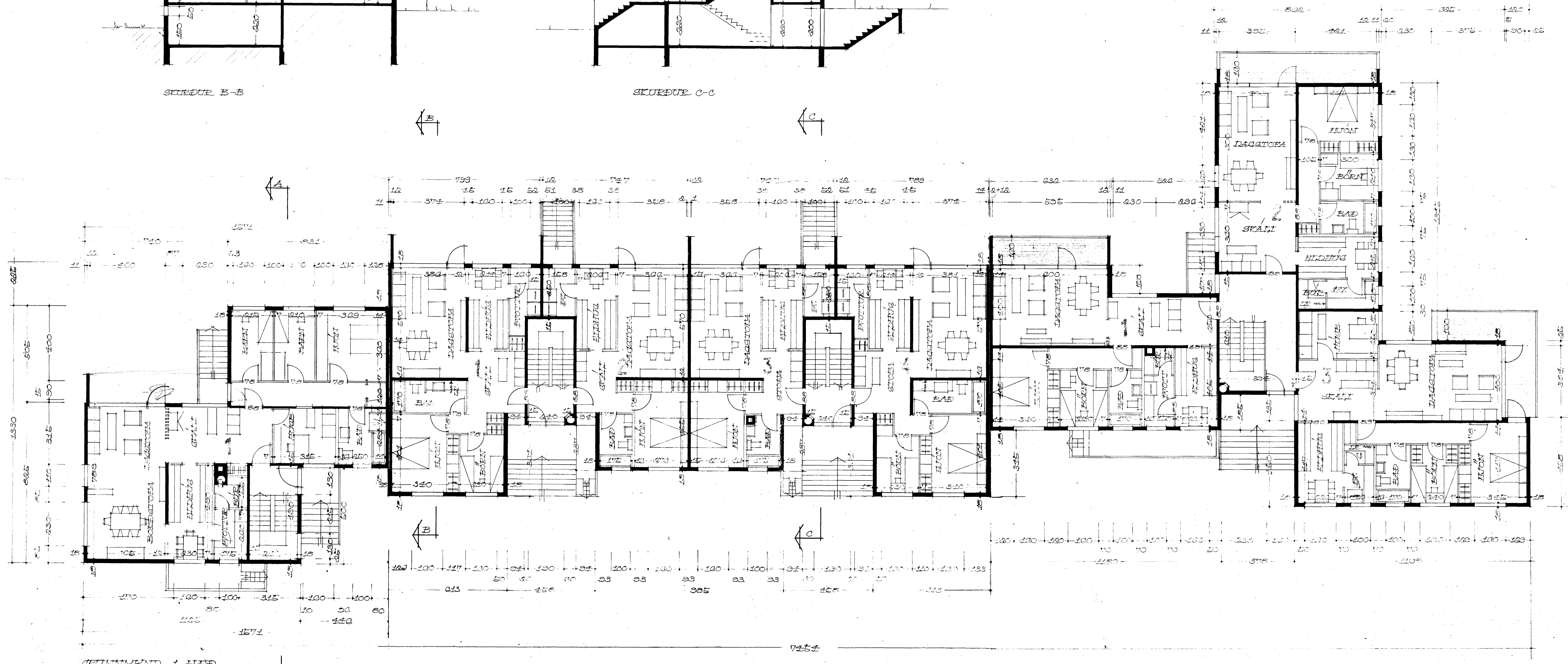
DRÖGGERÐ 1. HÆÐ
