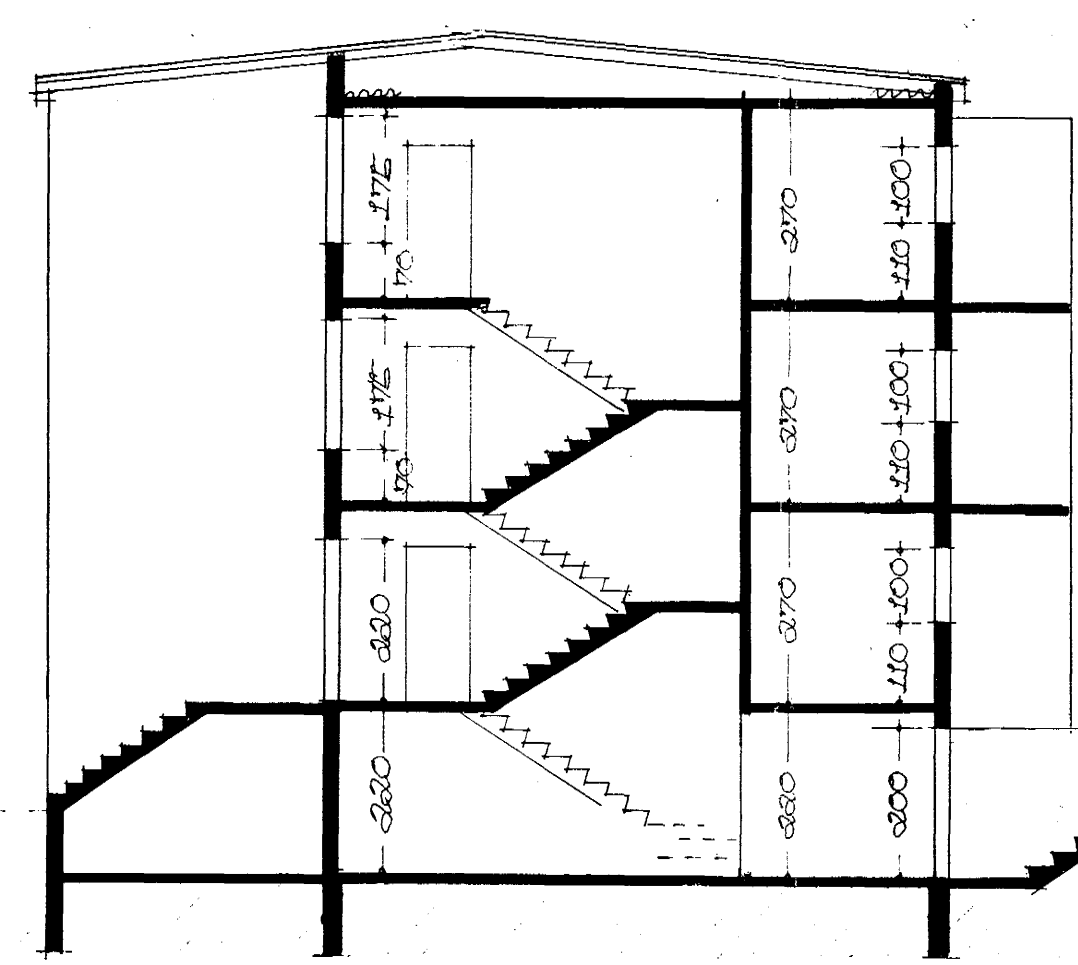
SKURÐUR C-C
