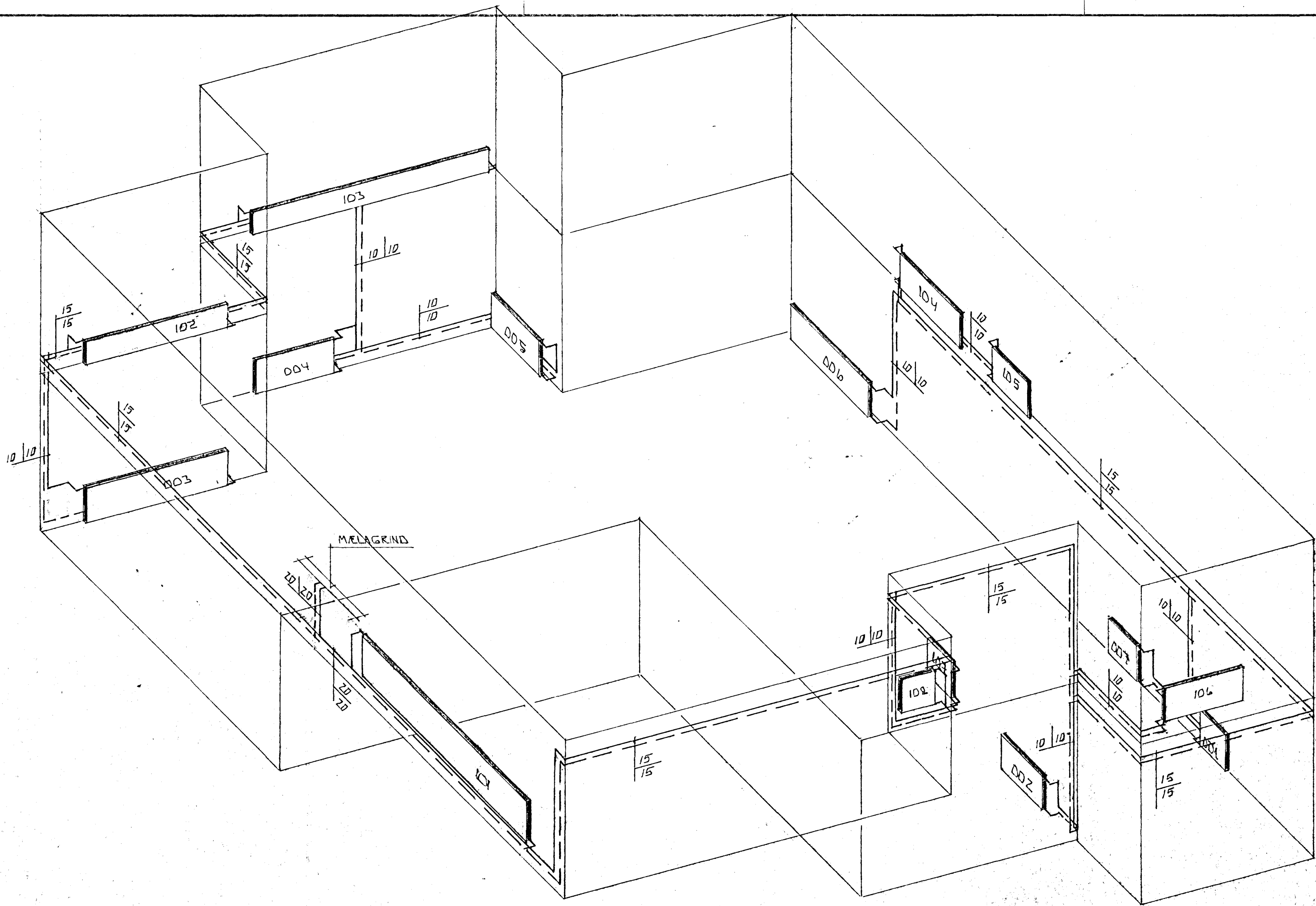
RÚMMYND HITALAGNA 1:50
