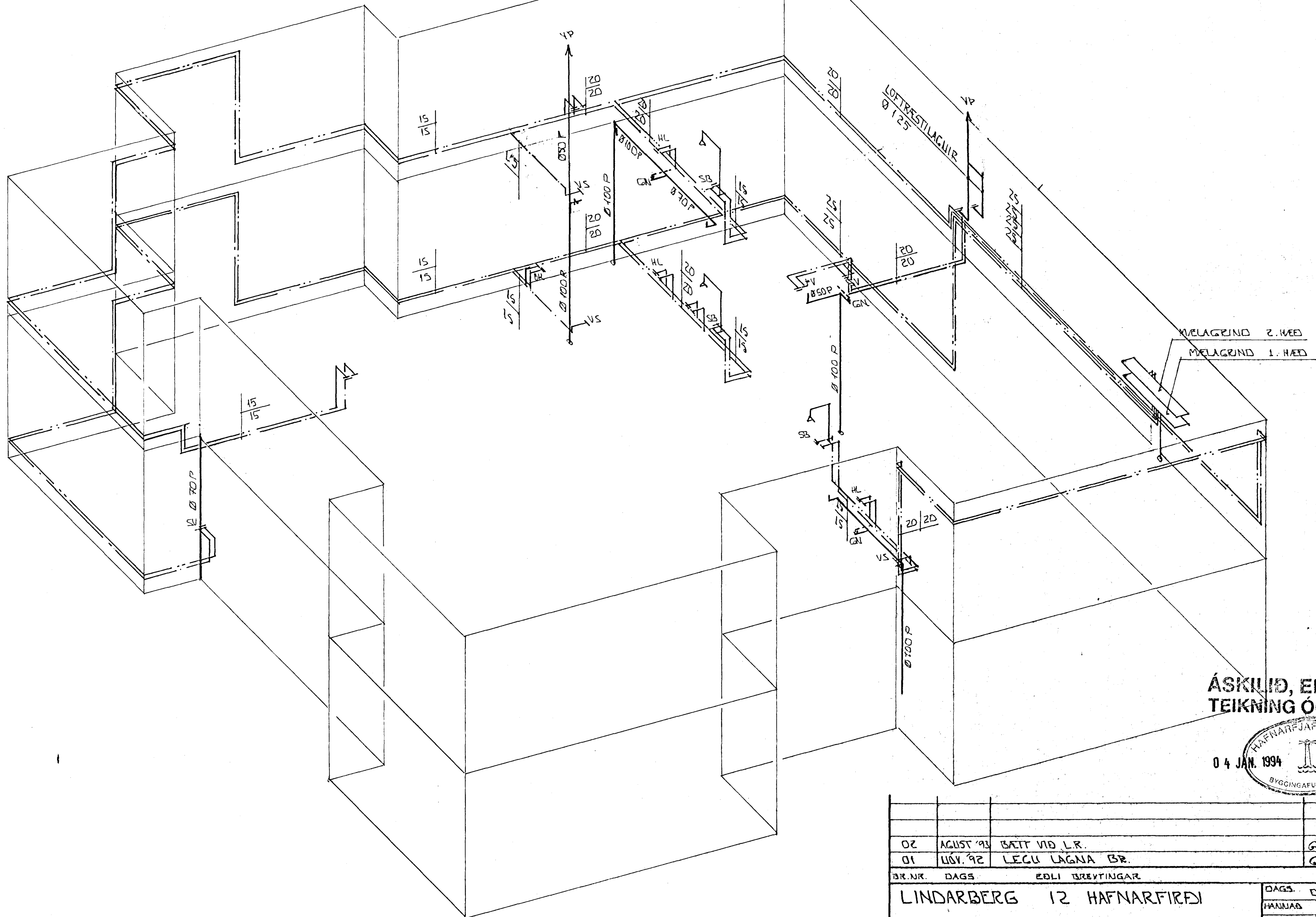
RÚMMYND VATNS- OG FRÆRENNSLISLAGNA 1:50
