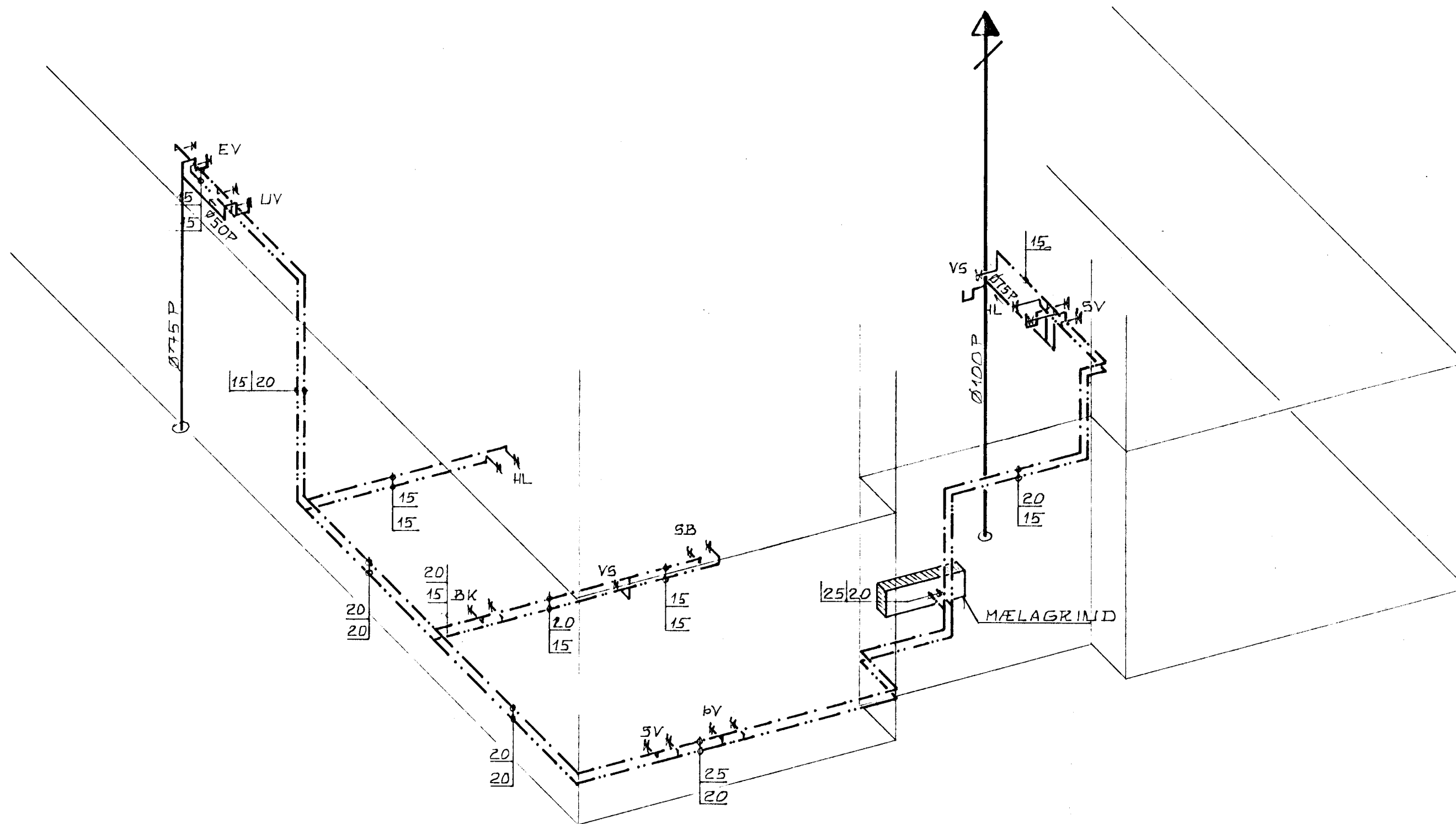
RÚMMYND VATNSLAGNA 1:50
