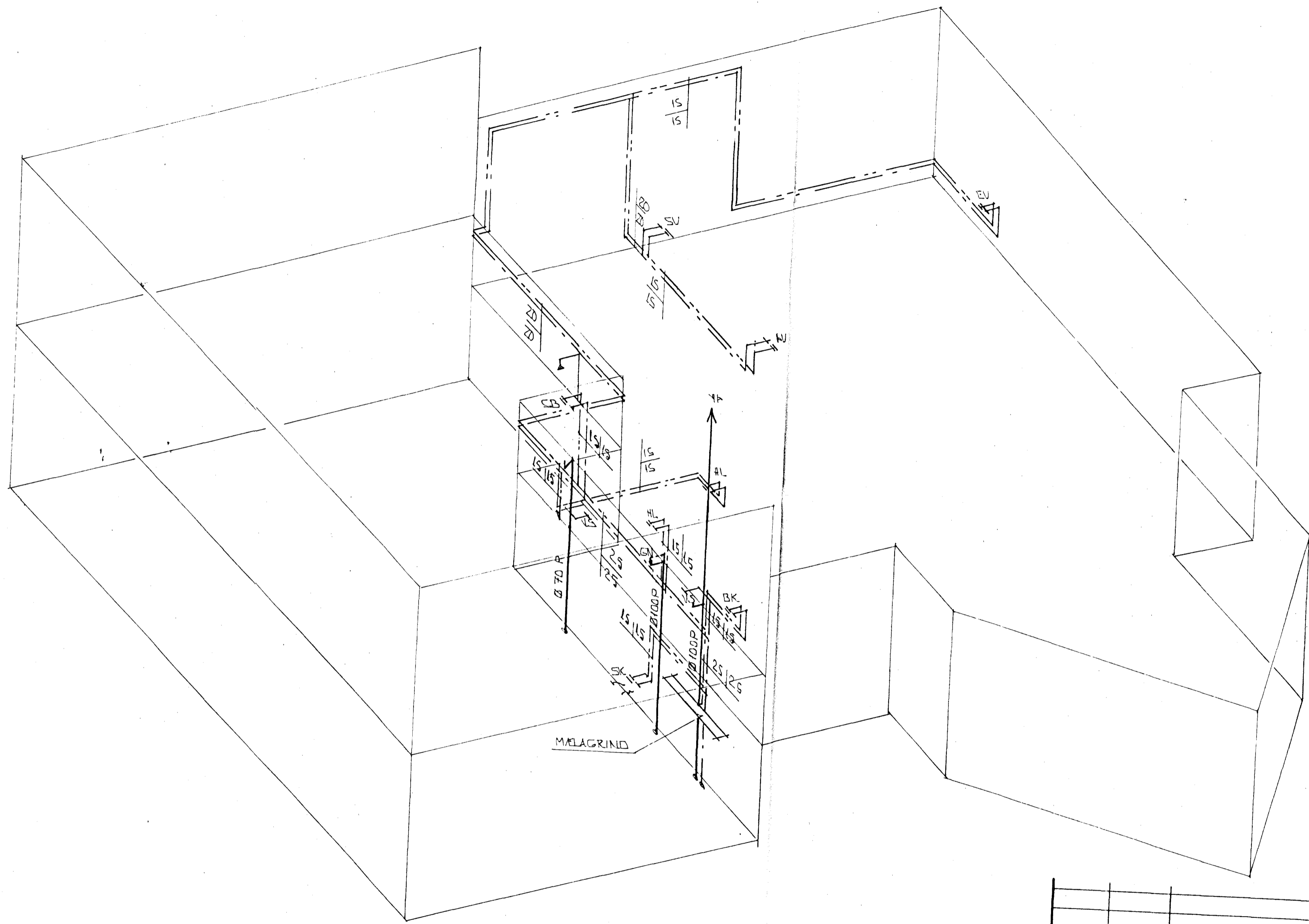
RÚMMYND VATNS- OG FRÆRENSLISLAGNA 1:50
