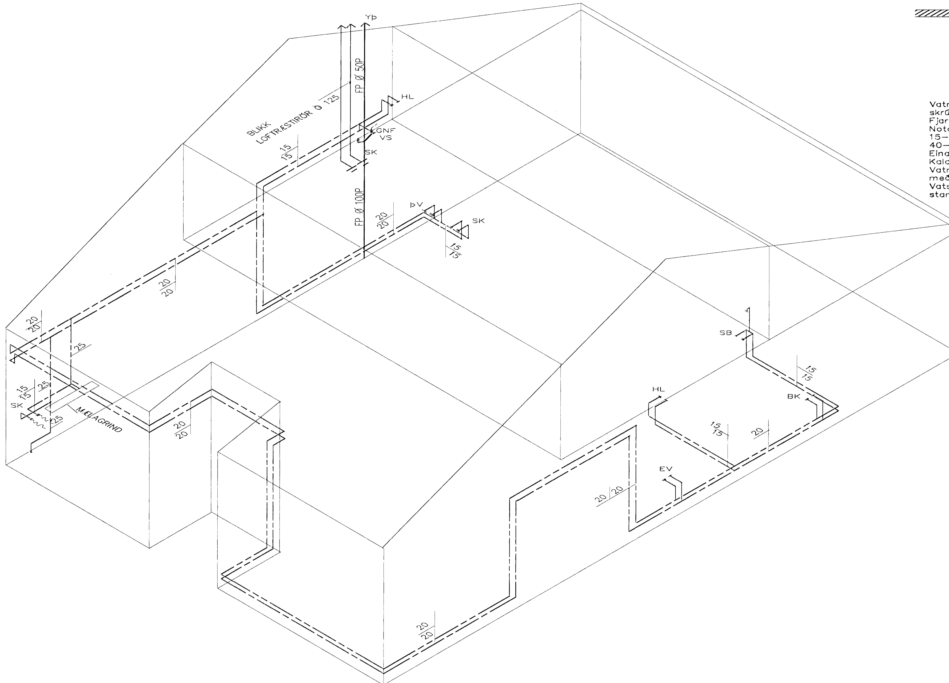
RÚMMYND VATNSLAGNA 1:50
