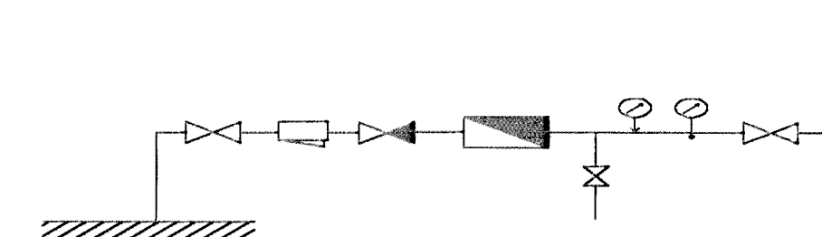
Inntak neysluvatn
