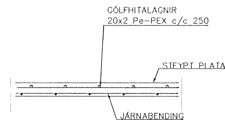
Gólfhiti, SNID, 1:20
