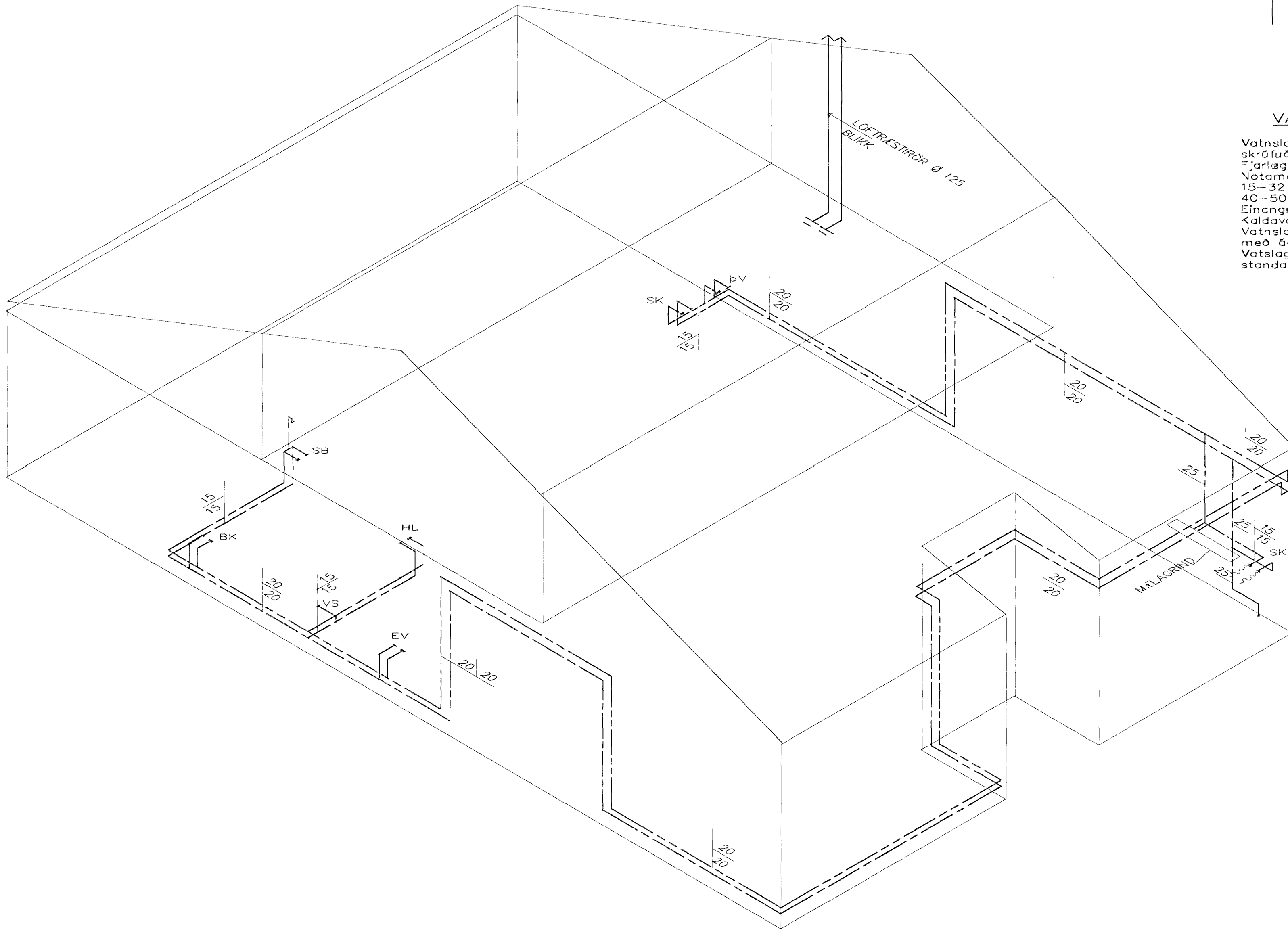
RÚMMYND VATNSLAGNA 1:50
