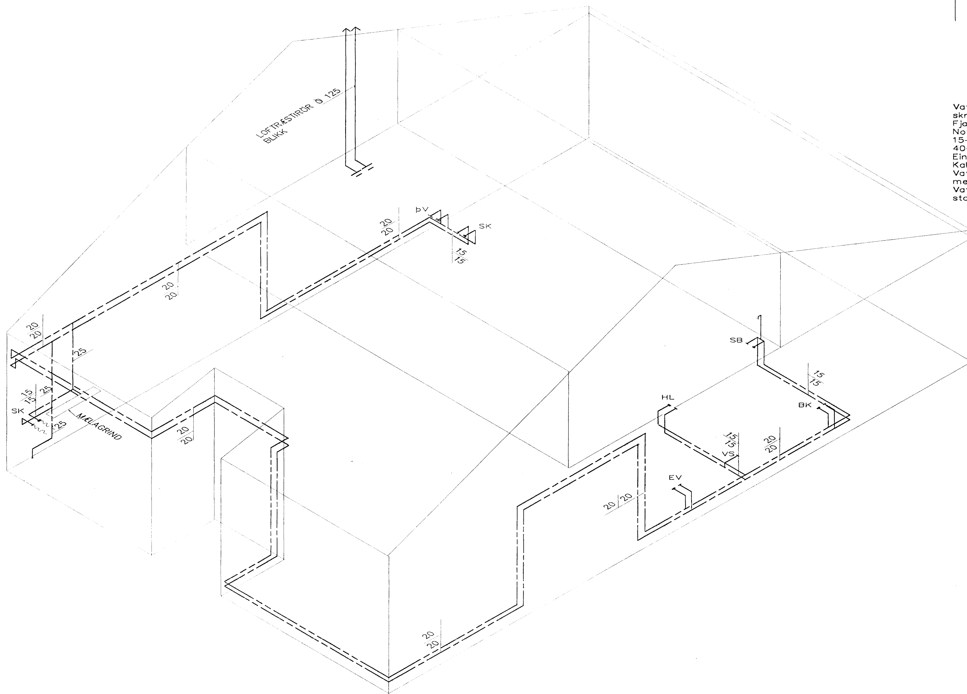
RÜMMYND VATNSLAGNA 1:50
