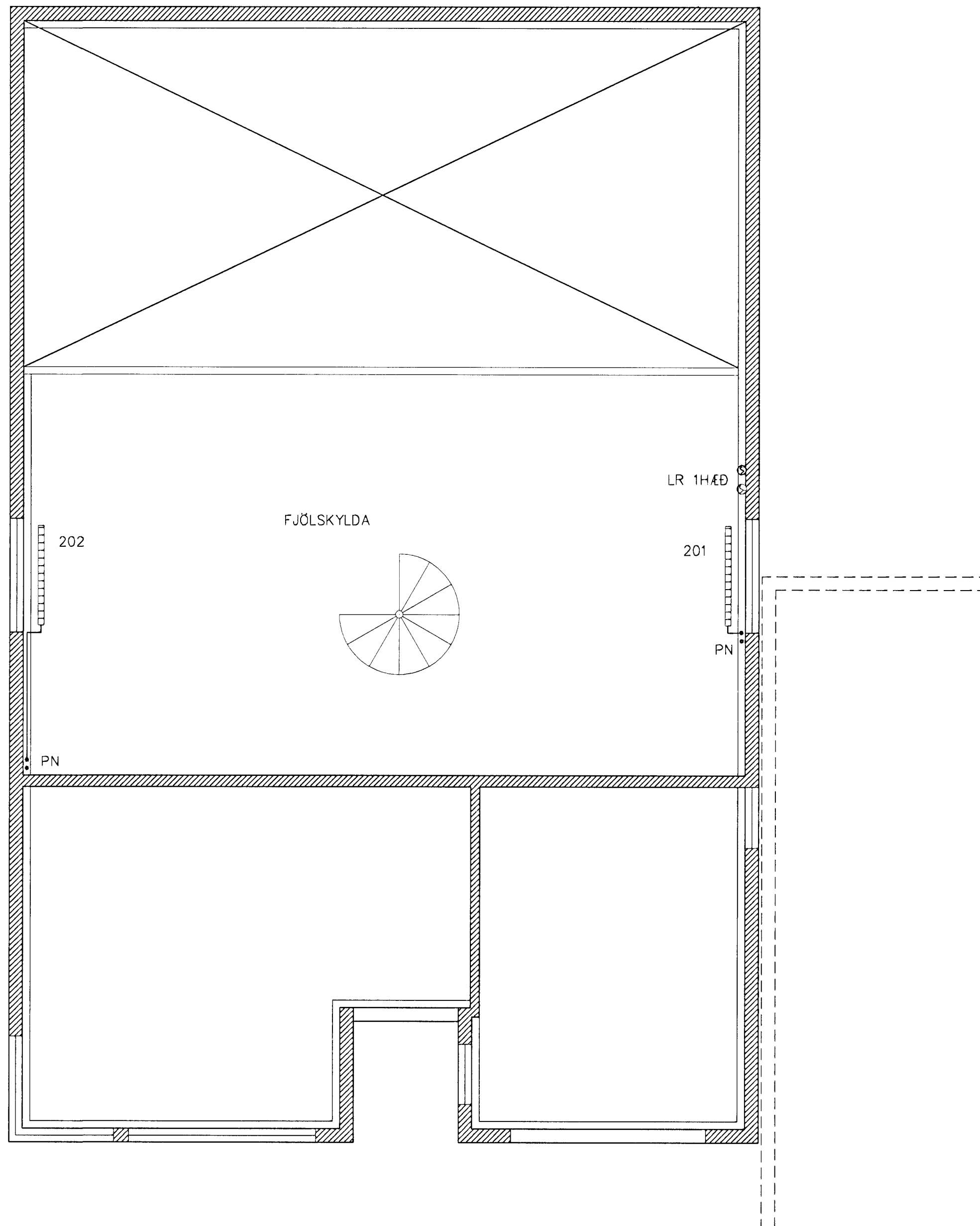
GRUNNMYND 2 HÆÐAR 1:50
